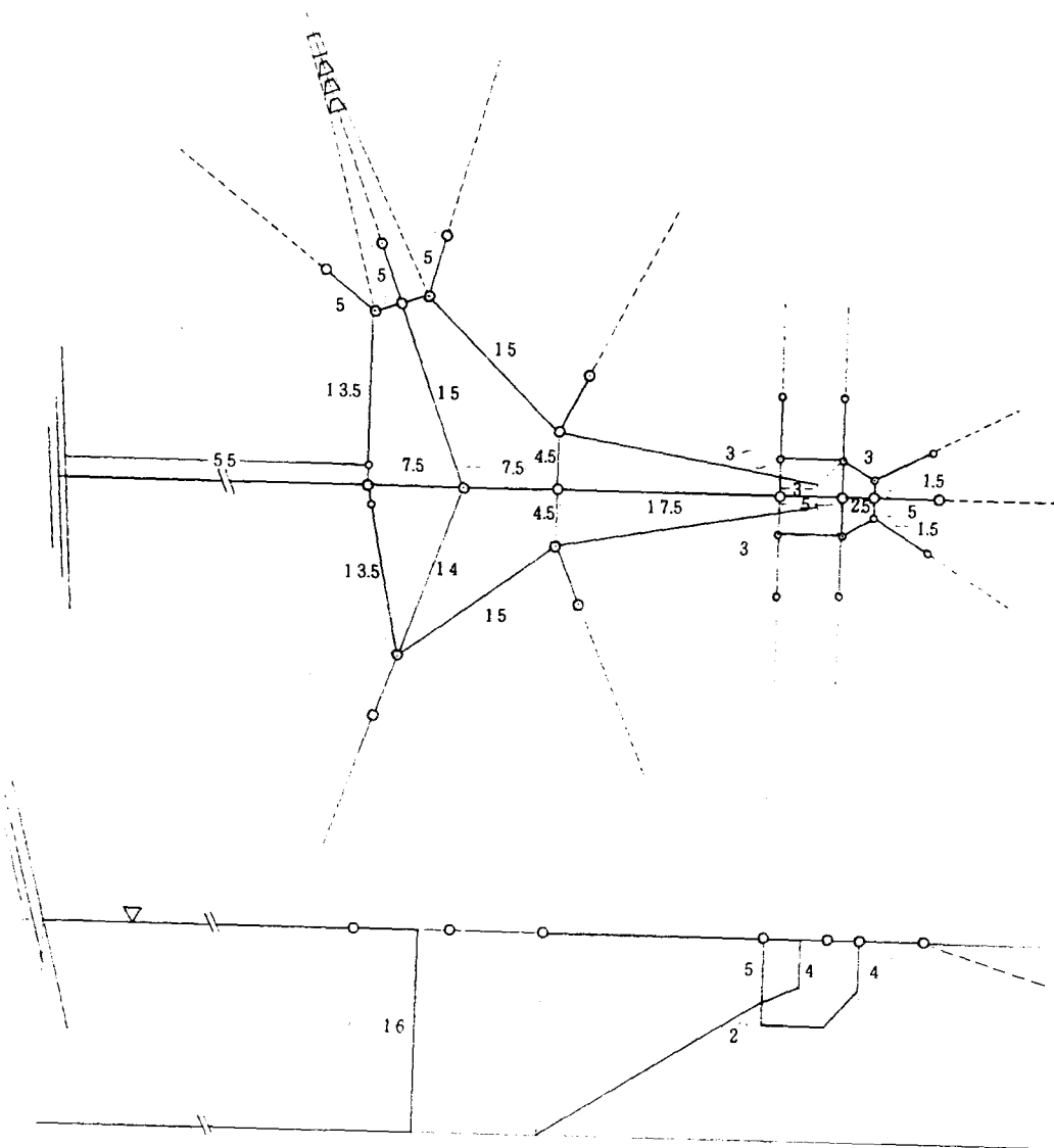
第1図 定置網（落網及び罟網）の側張と張立平面並びに断面の概要
