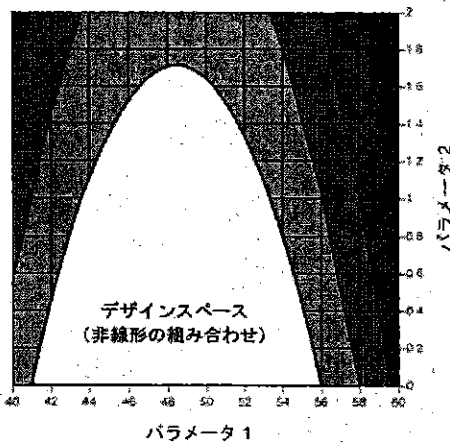
図1c: 造粒パラメータの非線形的な組み合わせで規定した、十分な溶出率 (80%超) をもたらず造粒パラメータのデザインスペース。
