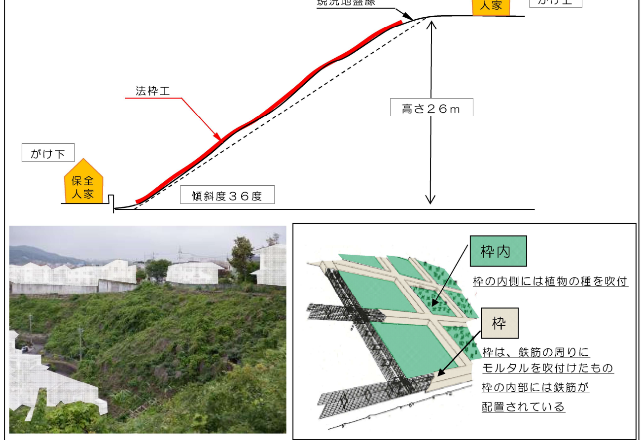
写真③ 急傾斜地崩壊防止施設（法枠工）の現在の状況
