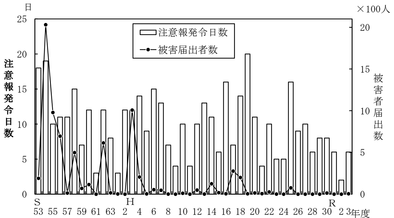
図9 光化学スモッグ注意報発令日数等の経年推移
