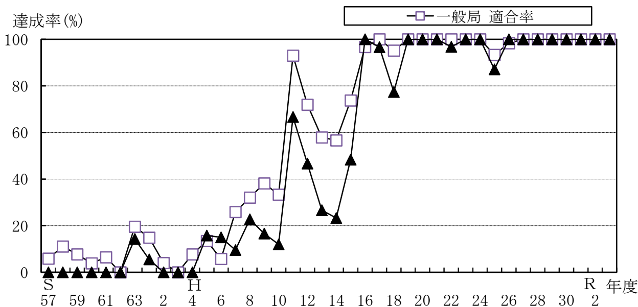
図 3 浮遊粒子状物質に係る環境基準 (長期的評価) 達成率の経年推移
