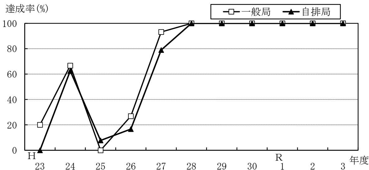
図 5 微小粒子状物質に係る環境基準達成率の経年推移
