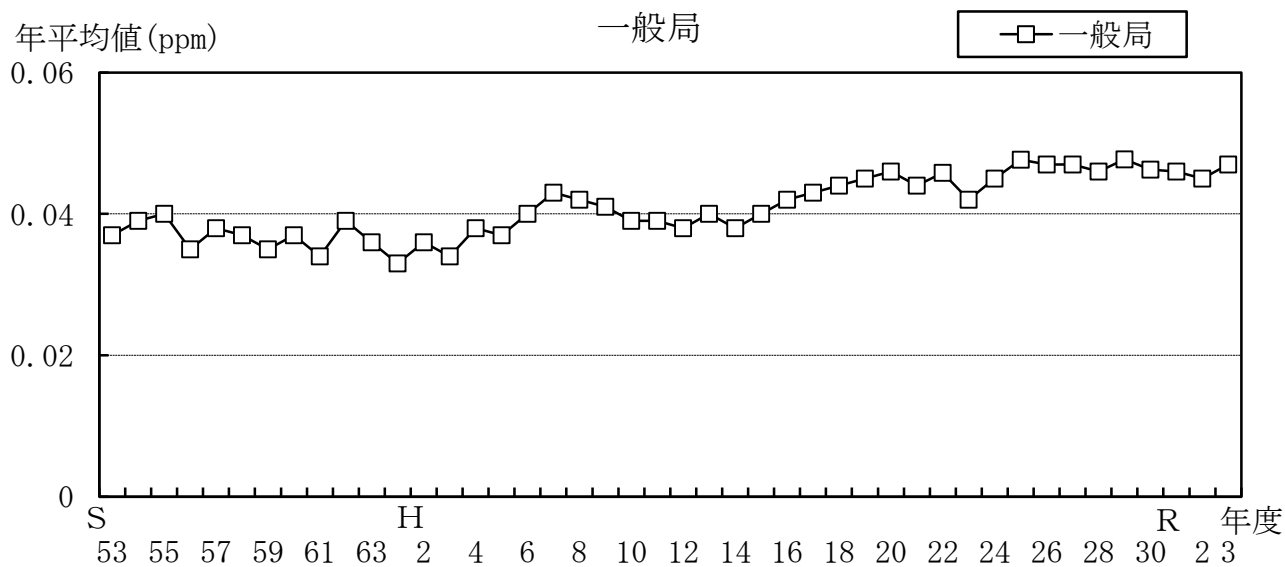
図10 光化学オキシダント濃度 (昼間の日最高1時間値の年平均値) の経年推移
