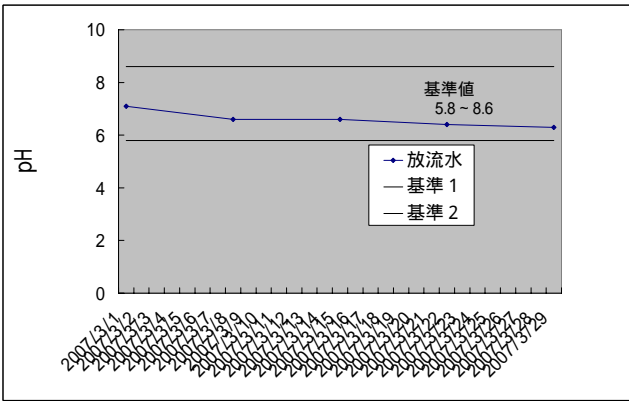
放流水と目標処理水質値の関係
