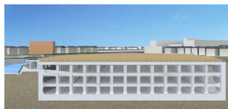
完成イメージ（断面）
