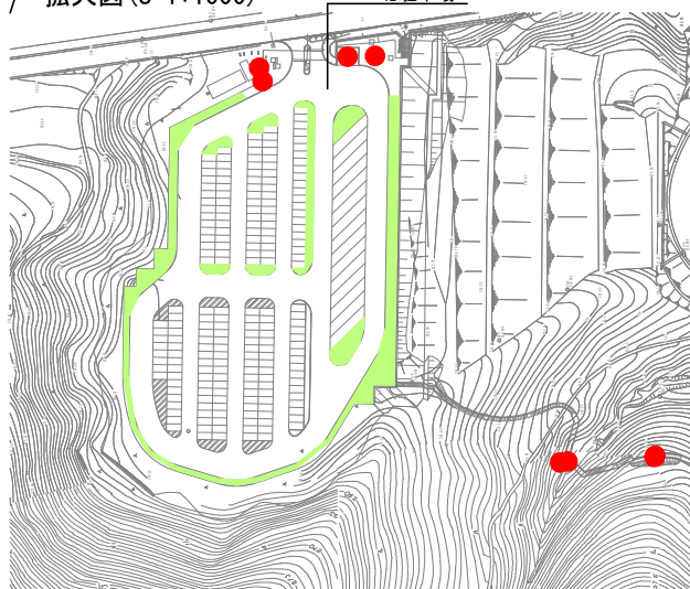
拡大図 (S=1:1000)
