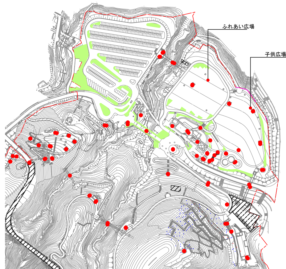
拡大図 (S=1:1500)
