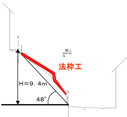
横断面図
