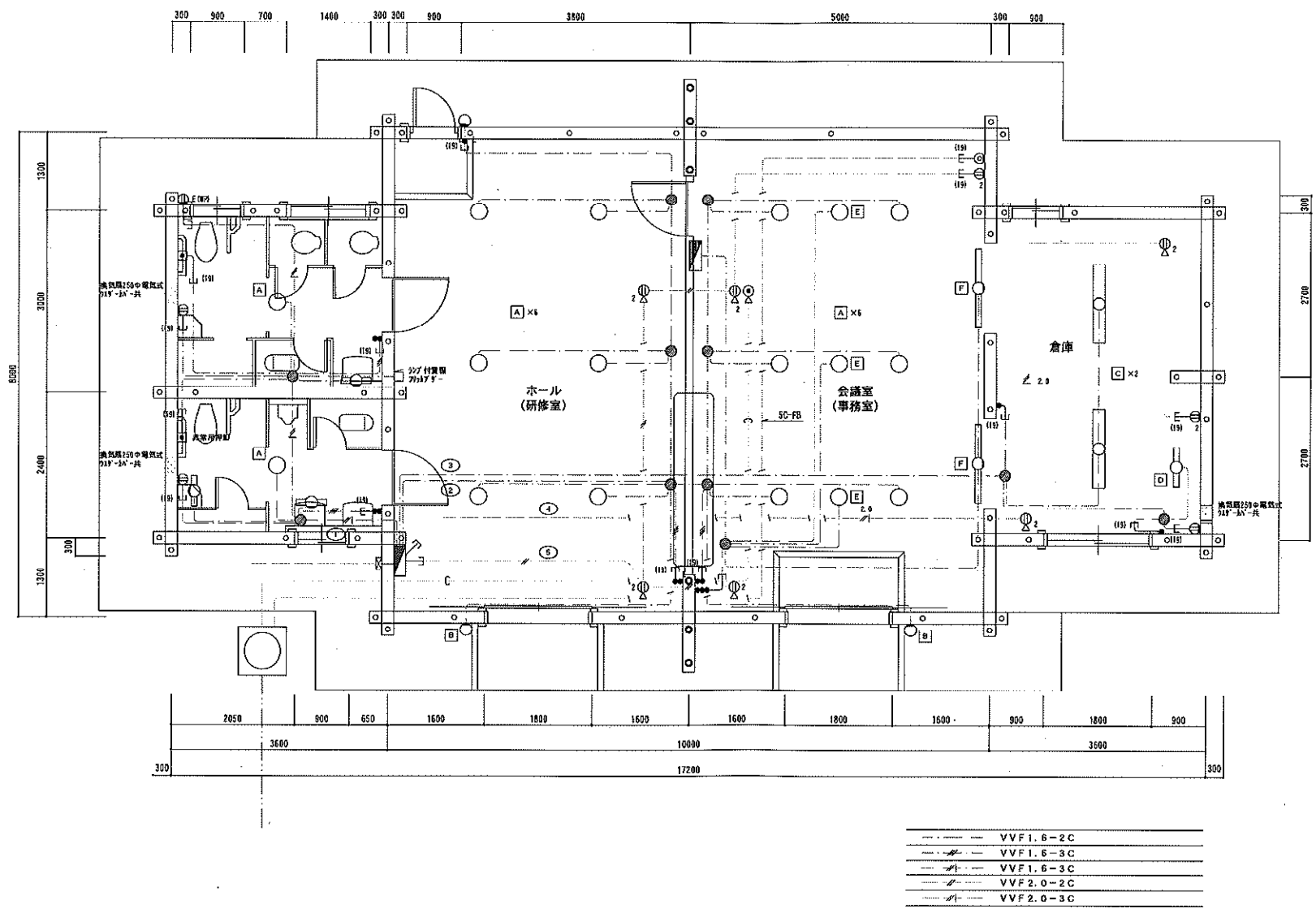
平面詳細図 S=1/50
