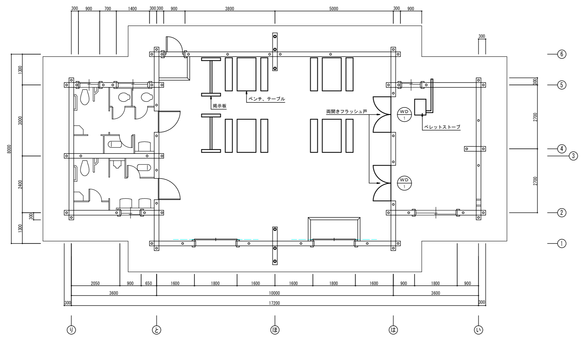
計画平面図 1/50
