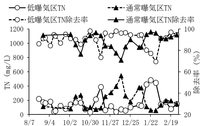
図2 処理水のTNとTN除去率の推移
