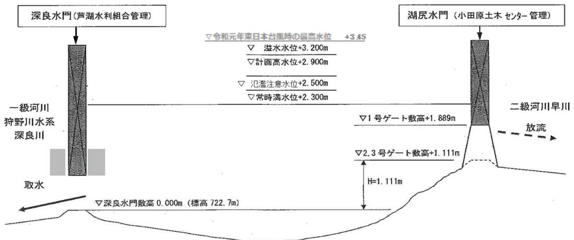
図 3 芦の湖水門関係イメージ図
