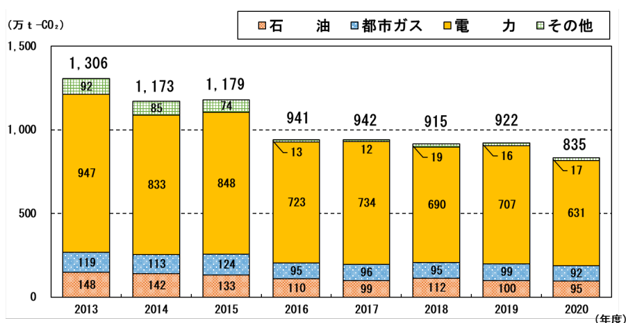
図2-3 CO 2 排出量の推移（業務部門）
