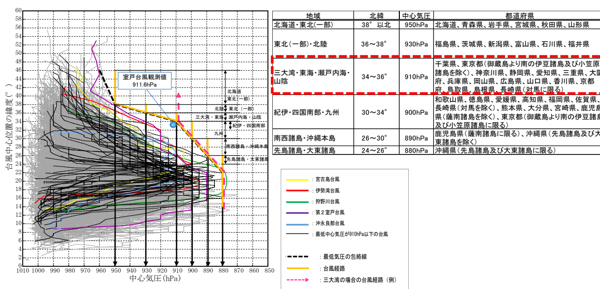
図－5 想定する台風の中心気圧
