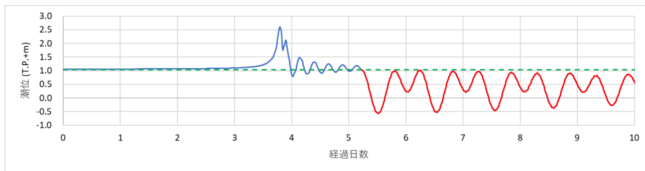
図－9 台風接近時からの経過時間と潮位
