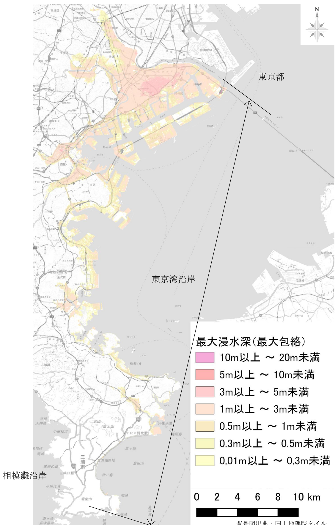
図－１４ 最大規模の高潮に対する最大の浸水区域及び浸水深
