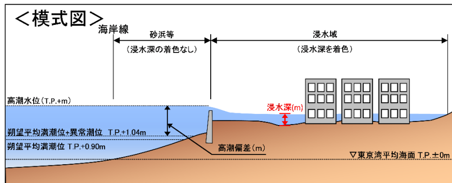
図－１ 高潮浸水想定区域図における用語の定義
