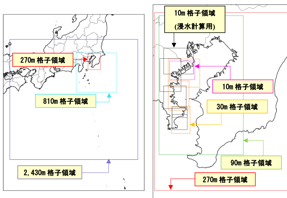
図－１１ 計算領域及び計算格子間隔
