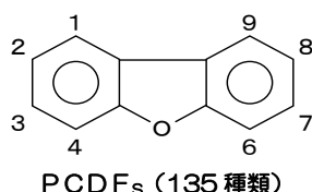
ダイオキシン類の構造式 (数字の付いた炭素原子に塩素原子または水素原子が結合)
