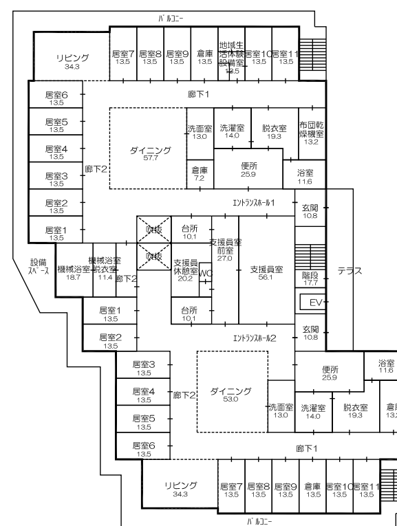
居住棟 2階平面図
