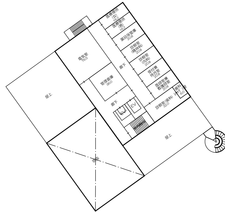
センター棟 3階平面図
