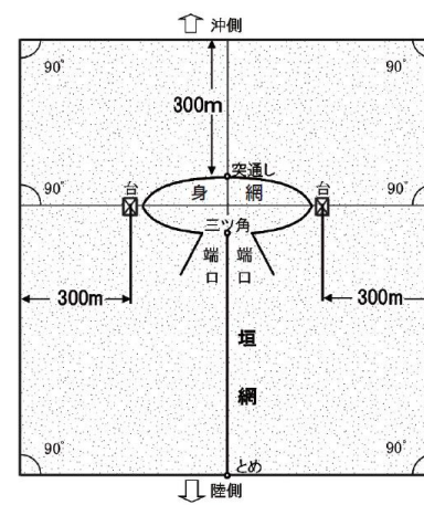
★いわし両口網
