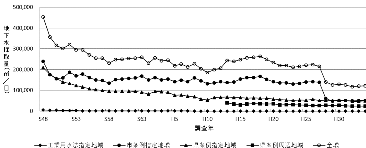
図4 地下水採取量の経年変化(全域)
