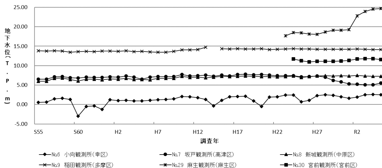
図6－2 地下水位の経年変化(川崎市幸区、高津区、中原区、多摩区、麻生区、宮前区)
