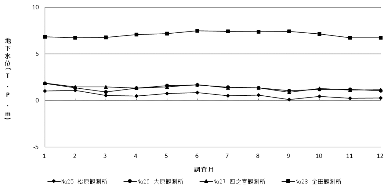
図5-5 令和5年地下水位の経月変化(平塚市)
