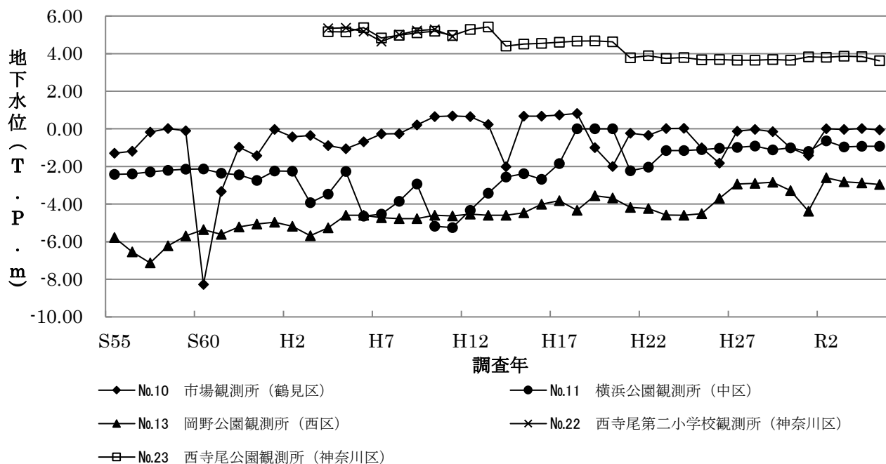
図6-4 地下水位の経年変化(横浜市鶴見区、神奈川区、西区、中区)
