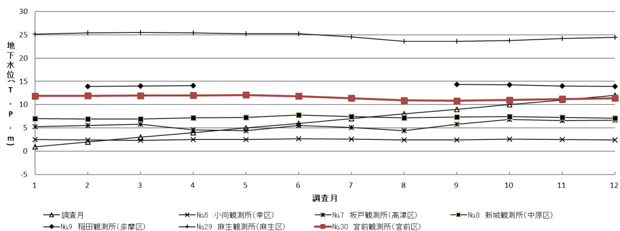
図5-2 令和5年地下水位の経月変化(川崎市幸区、高津区、中原区、多摩区、麻生区、宮前区)
