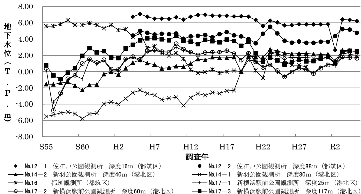
図6-3 地下水位の経年変化(横浜市都筑区、港北区)
