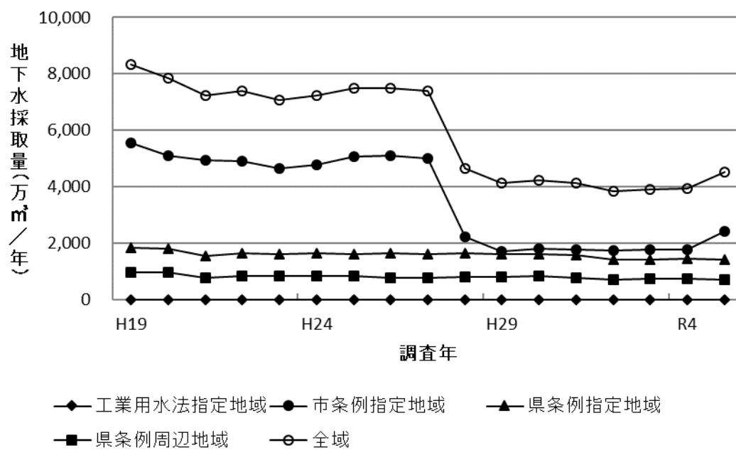
図3 地下水採取量の経年変化(全域)
