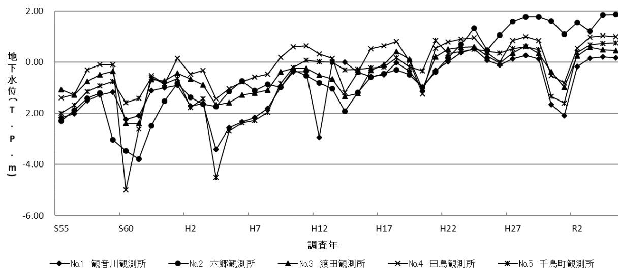
図6－1 地下水位の経年変化(川崎市川崎区)
