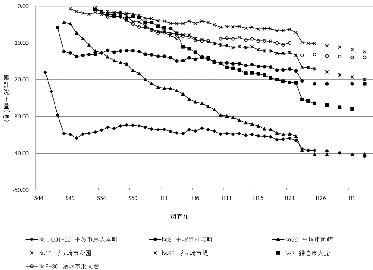
図3-4 主要水準点の沈下状況の経年変化 県央・湘南地域(1)
