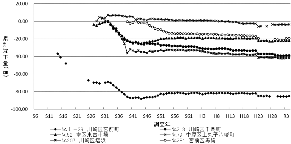
図3-3 主要水準点の沈下状況の経年変化 川崎地域
