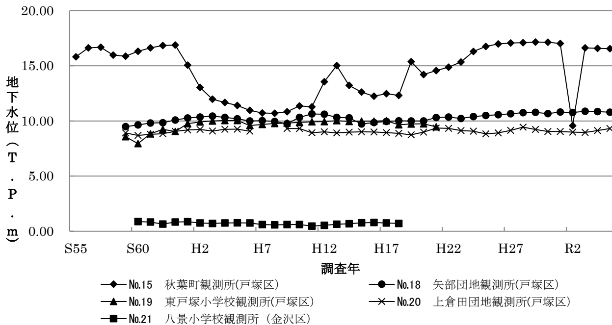
図6-5 地下水位の経年変化(横浜市戸塚区、金沢区)
