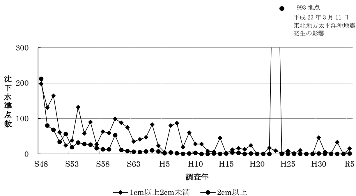
図1 1cm以上沈下水準点数の経年変化(全域)
