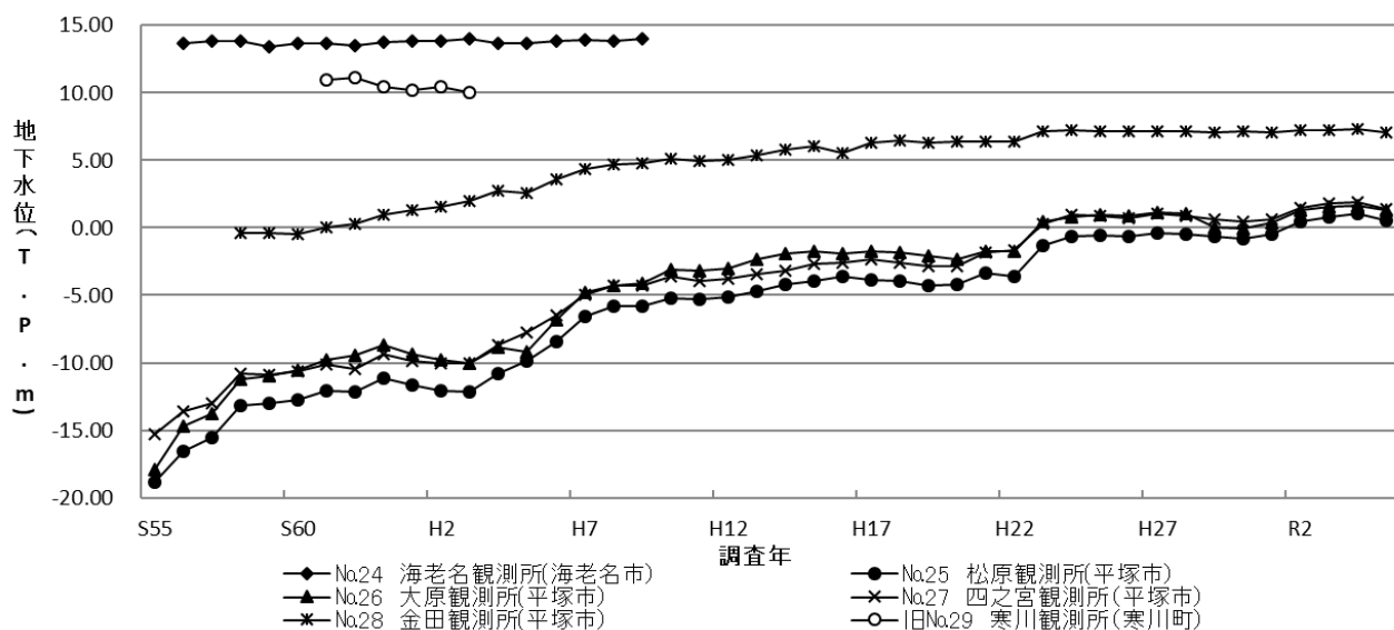
図6-6 地下水位の経年変化(平塚市、海老名市、寒川町)
