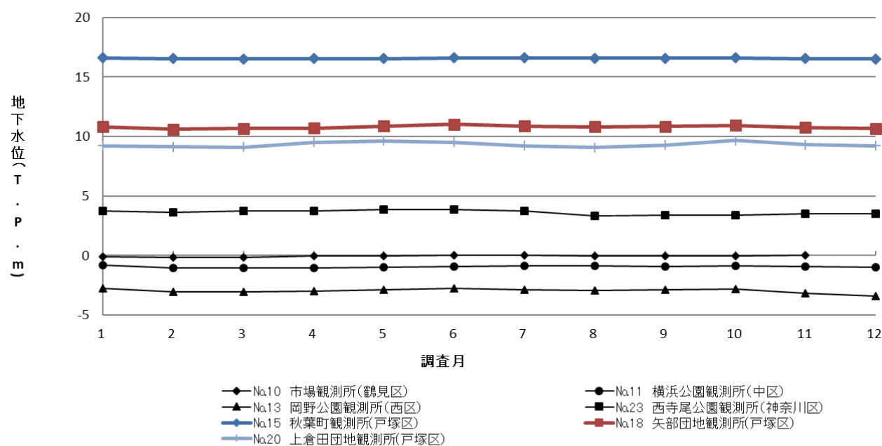
図5-4 令和5年地下水位の経月変化(横浜市鶴見区、神奈川区、西区、中区、戸塚区、金沢区)
