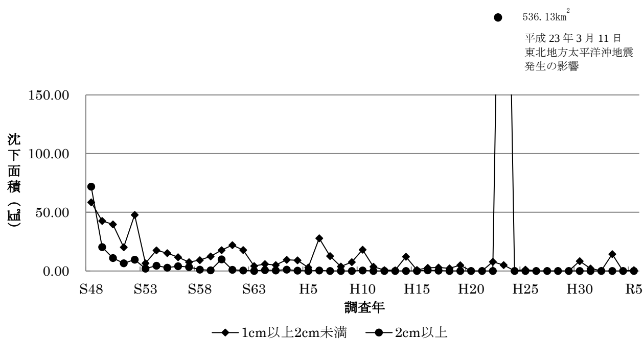
図2 1cm以上沈下面積の経年変化(全域)
