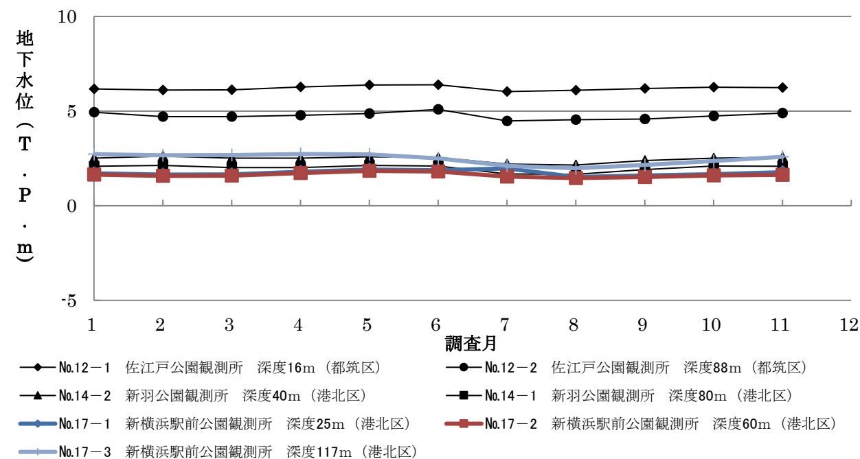
図5-3 令和5年地下水位の経月変化(横浜市都筑区、港北区)
