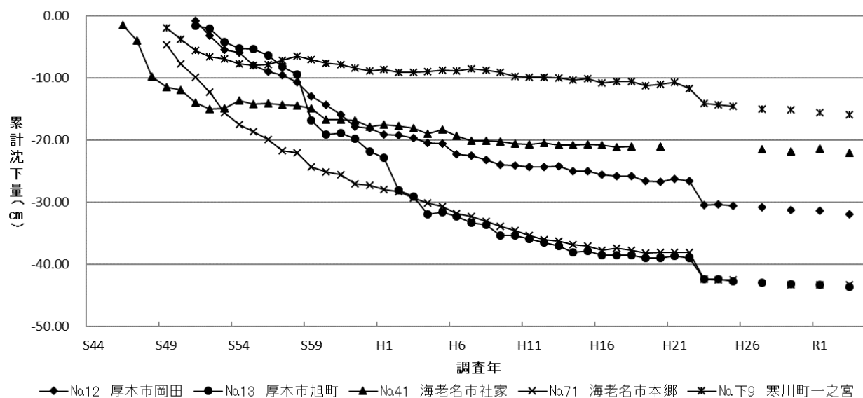
図3-5 主要水準点の沈下状況の経年変化 県央・湘南地域(2)
