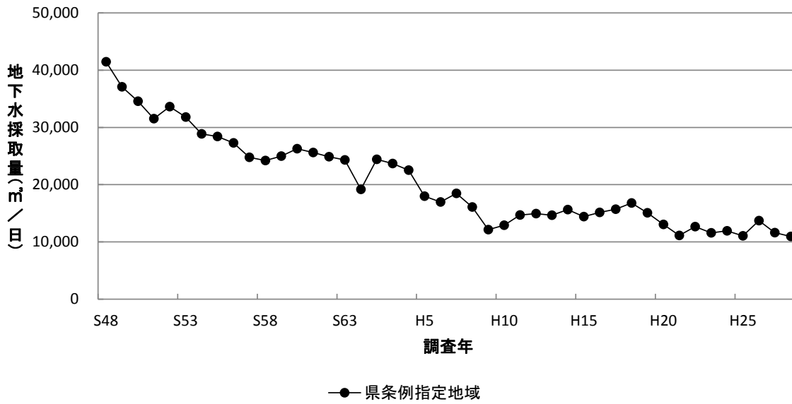
図1-4 地下水採取量の経年変化(茅ヶ崎市)
