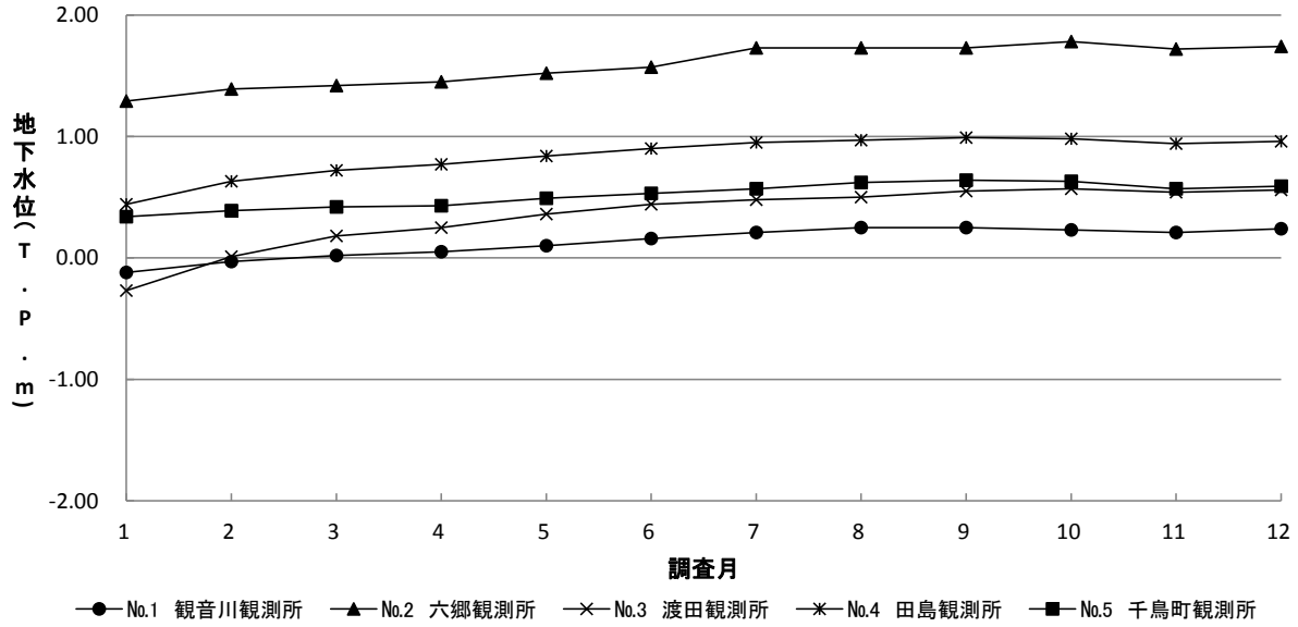
図7-7 平成27年地下水位の経月変化(川崎市川崎区)
