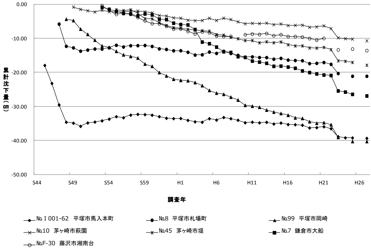
図5-1 主要水準点の沈下状況の経年変化 県央・湘南地域(1)
