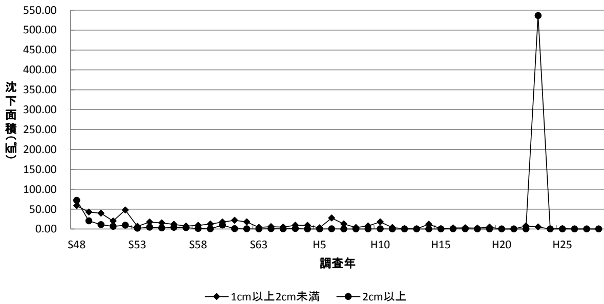
図2-2 1cm以上沈下面積の経年変化(全域)
