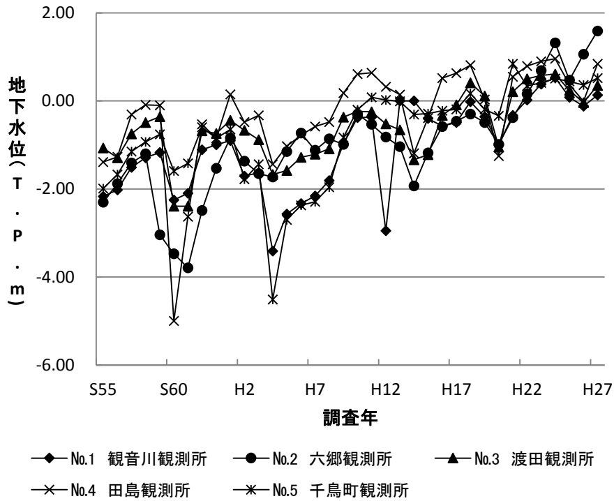
図7-1 地下水位の経年変化(川崎市川崎区)
