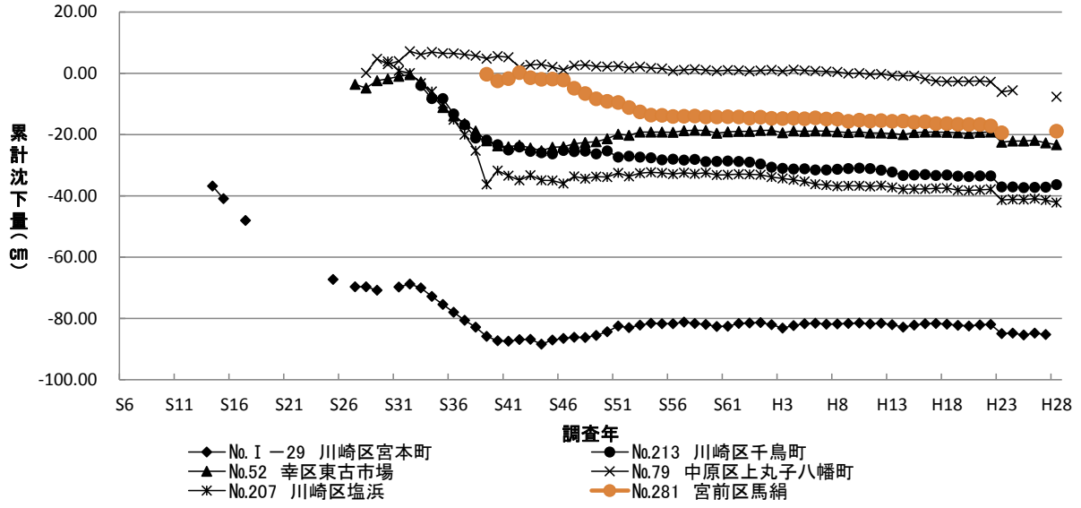
図4 主要水準点の沈下状況の経年変化 川崎地域
