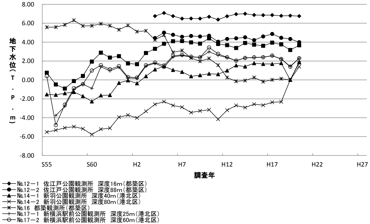
図7-3 地下水位の経年変化(横浜市都築区、港北区)
