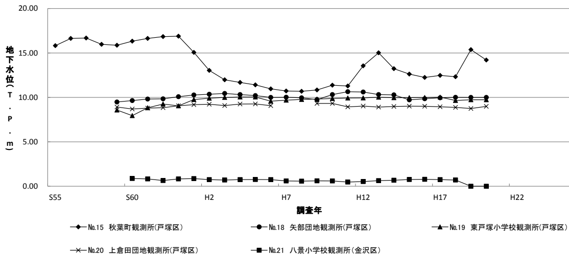
図7-5 地下水位の経年変化(横浜市戸塚区、金沢区)
