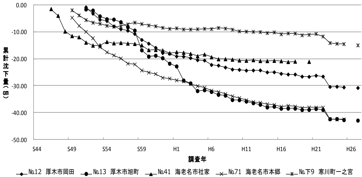
図5-2 主要水準点の沈下状況の経年変化 県央・湘南地域(2)
