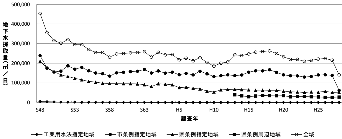
図1-10 地下水採取量の経年変化(全域)
