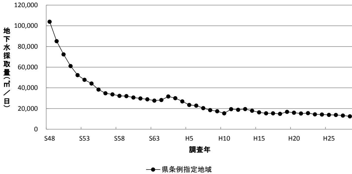
図1-3 地下水採取量の経年変化(平塚市)
