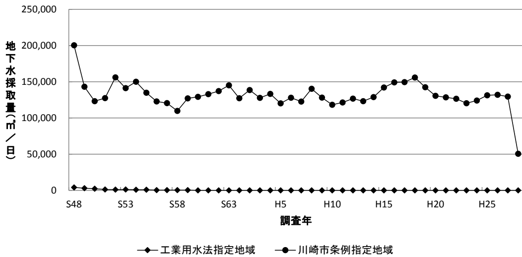
図1-2 地下水採取量の経年変化(川崎市)
