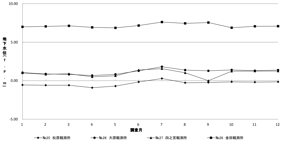
図7-9 平成27年地下水位の経月変化(平塚市)
