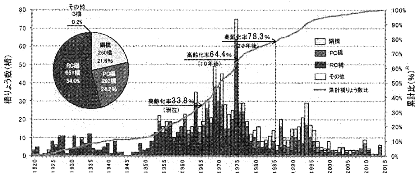
図2-1 橋種別建設年次分布（橋数ベース）
