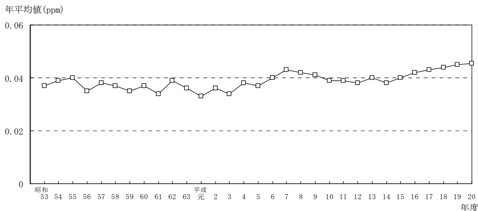
図6 光化学オキシダント濃度 (昼間の日最高1時間値の年平均値) の経年推移
