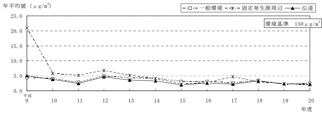
図 14 ジクロロメタンの地域分類ごとの年平均値の経年推移
