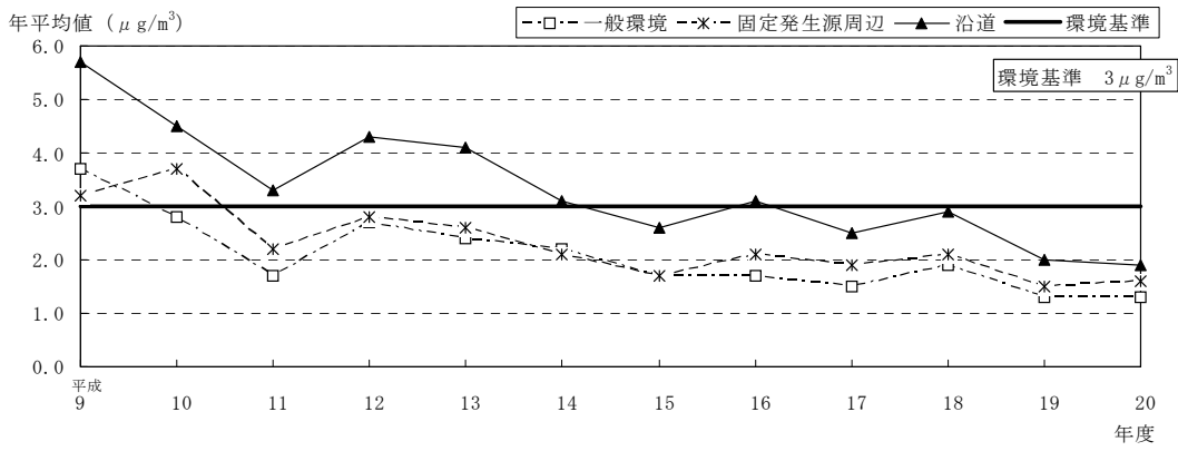
図 11 ベンゼンの地域分類ごとの年平均値の経年推移
