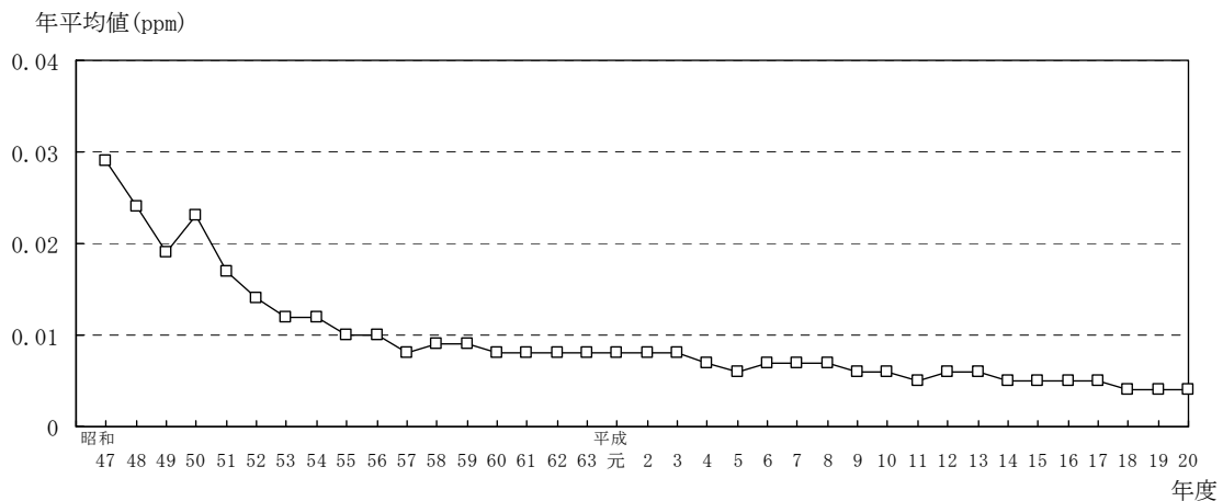
図8 二酸化硫黄濃度の年平均値の経年推移
