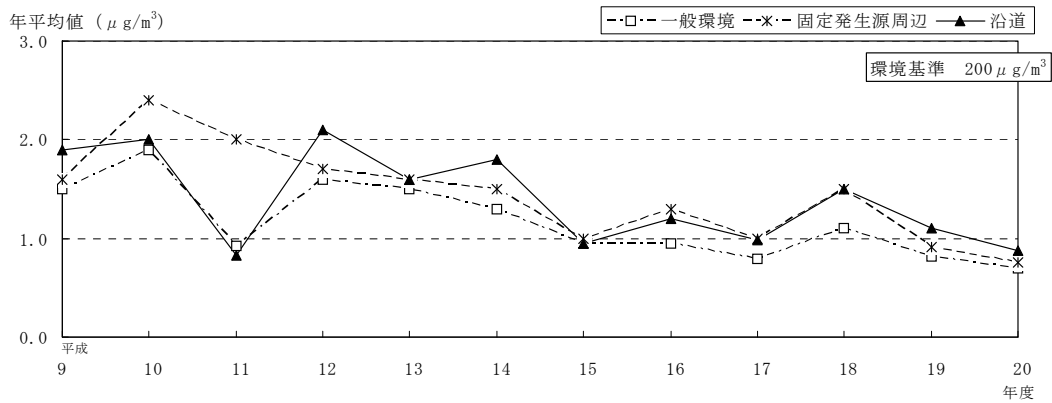
図 12 トリクロロエチレンの地域分類ごとの年平均値の経年推移
