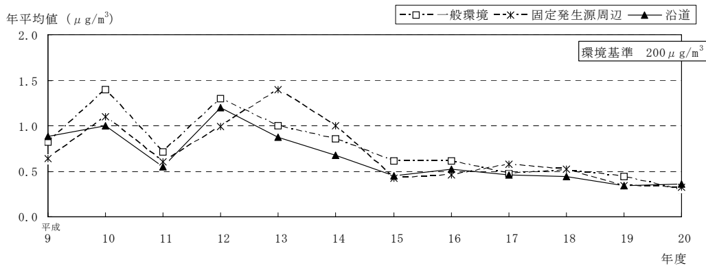
図 13 テトラクロロエチレンの地域分類ごとの年平均値の経年推移
