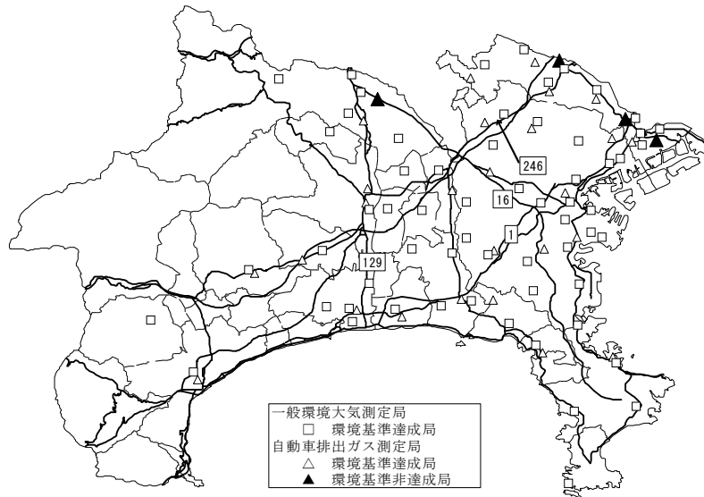
図2 各測定局の二酸化窒素に係る環境基準達成状況
