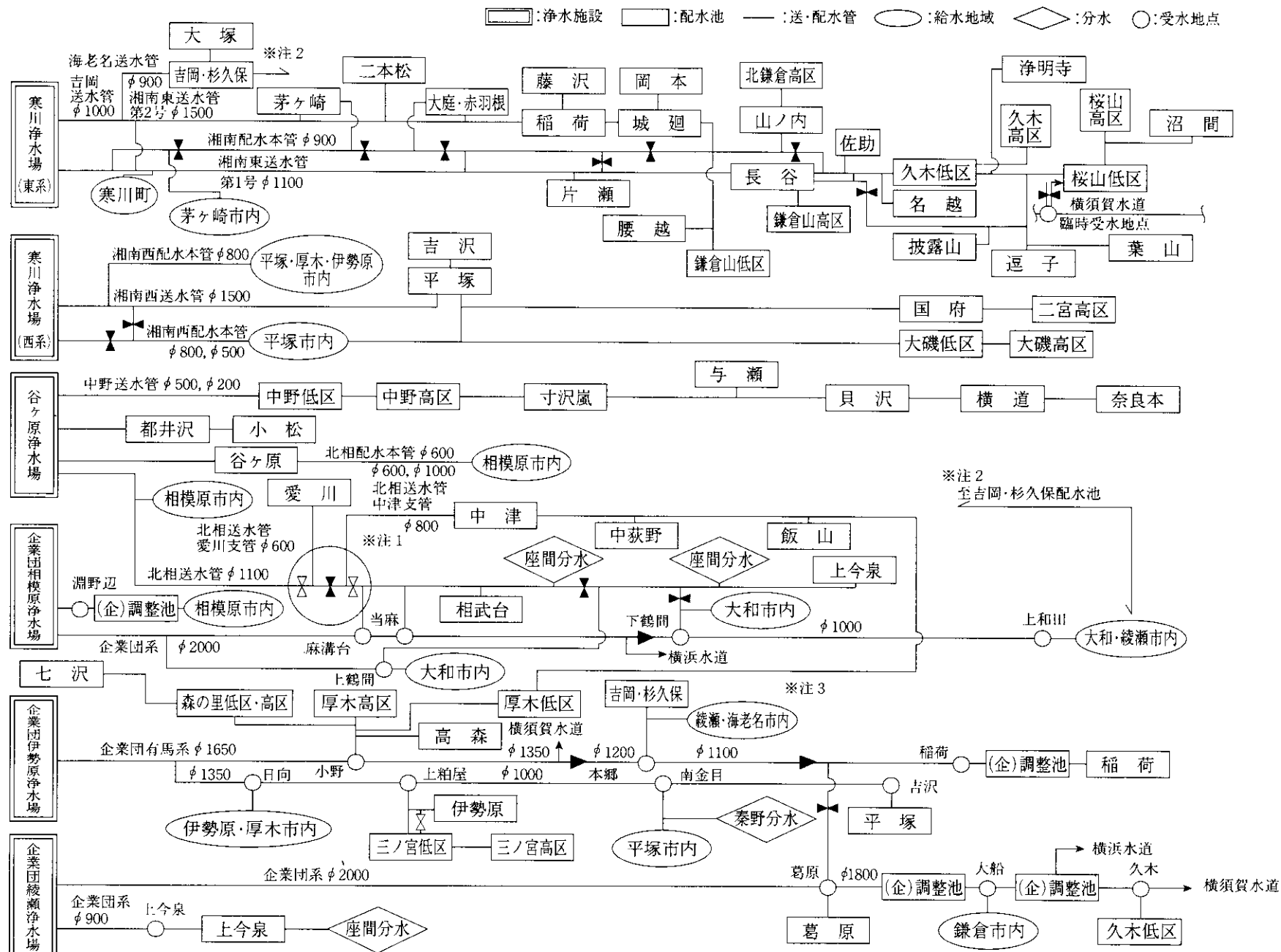
(7) 主配水系統図
