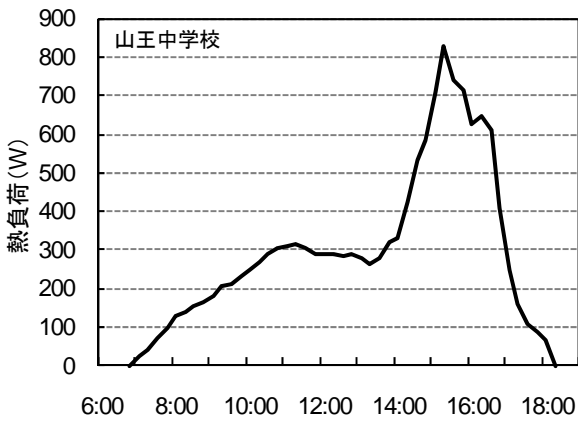
図10 壁面緑化により除去された熱負荷
