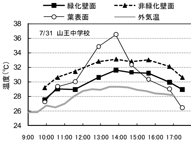
図4 日中の表面温度と外気温の推移
