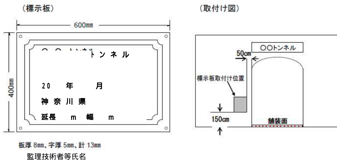
図8-6-2 標示板の刻示標準図
