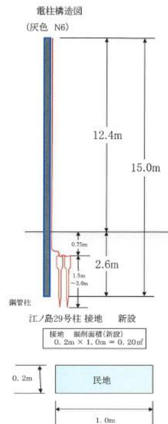
設計図
