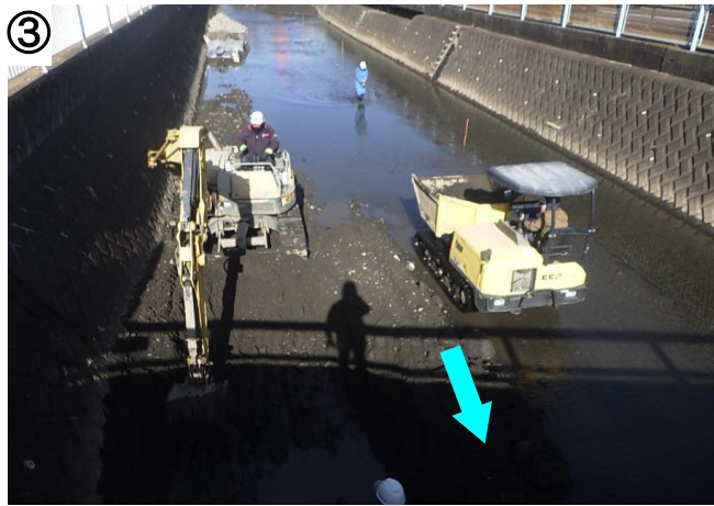
③の写真では、右岸側に根固工を施工するために、河床を掘削しています。
