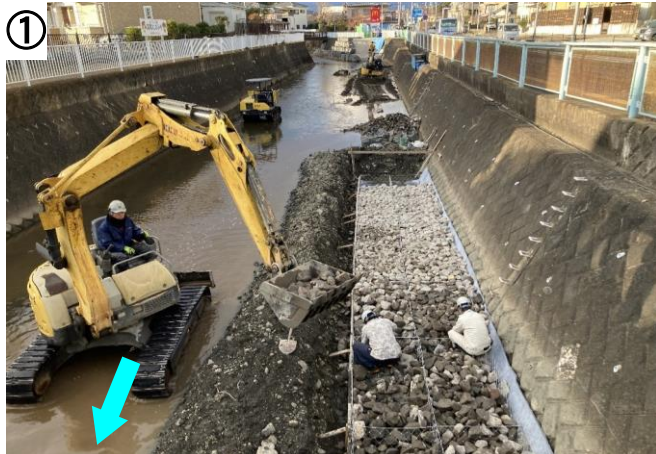
①の写真は、左岸側の根固工の施工状況で、かごマットという鋼製のかごに割栗石を敷詰めている様子です。
