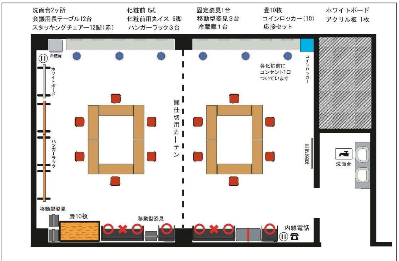
第7楽屋(2F) 備品配置図 定員24名
