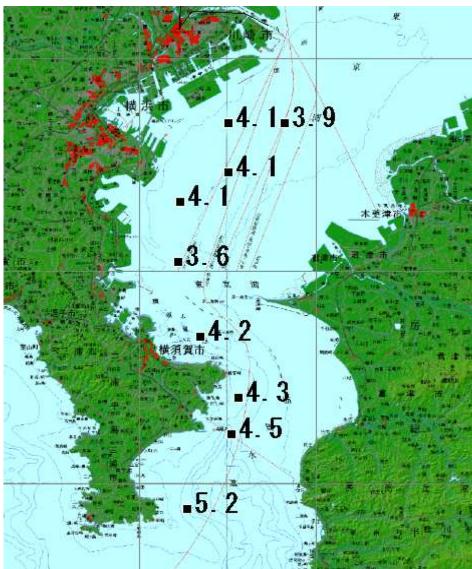
底層の溶存酸素量 (ml/l)
