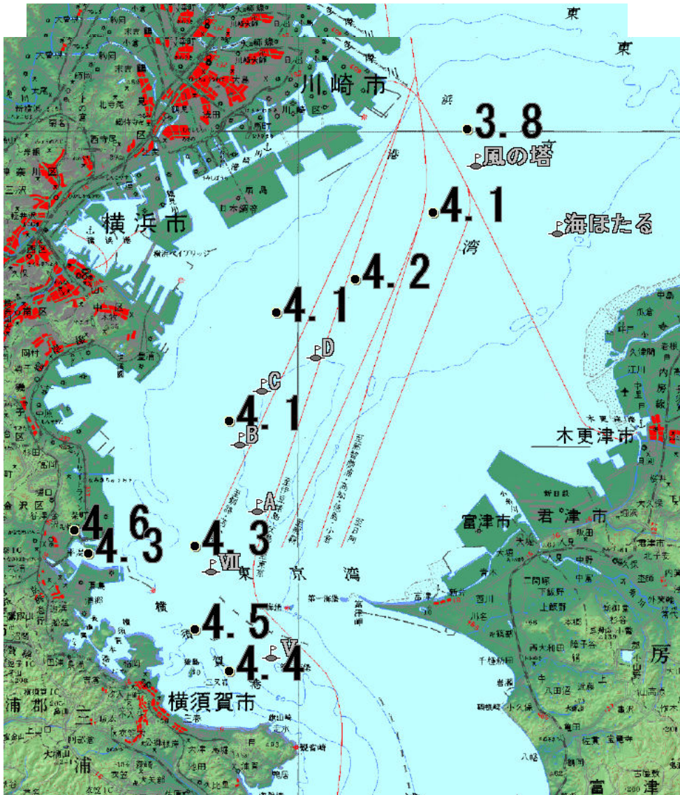
底層の溶存酸素量(ml/l)
