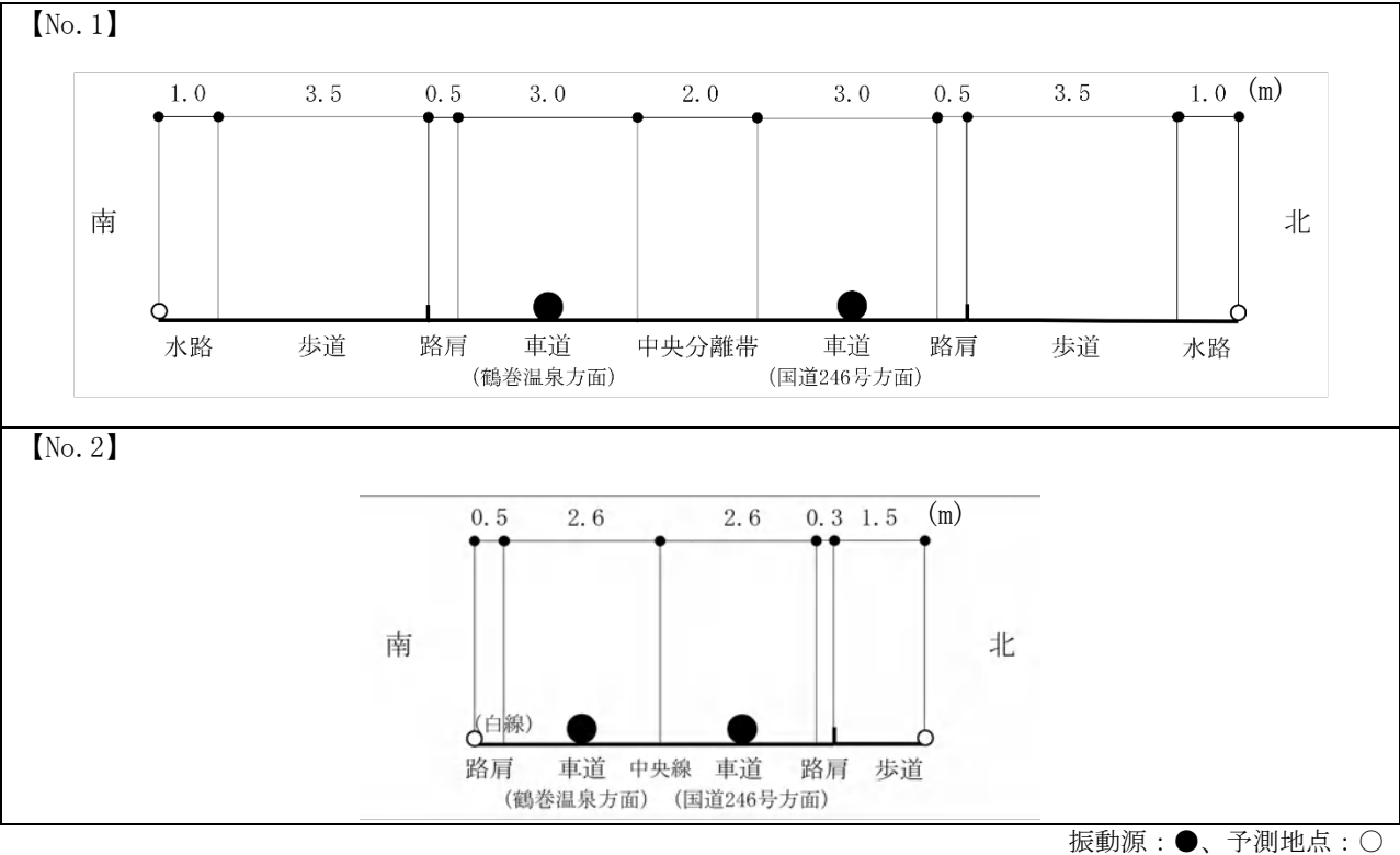
図 5-2-4-4 道路条件及び振動源の位置
