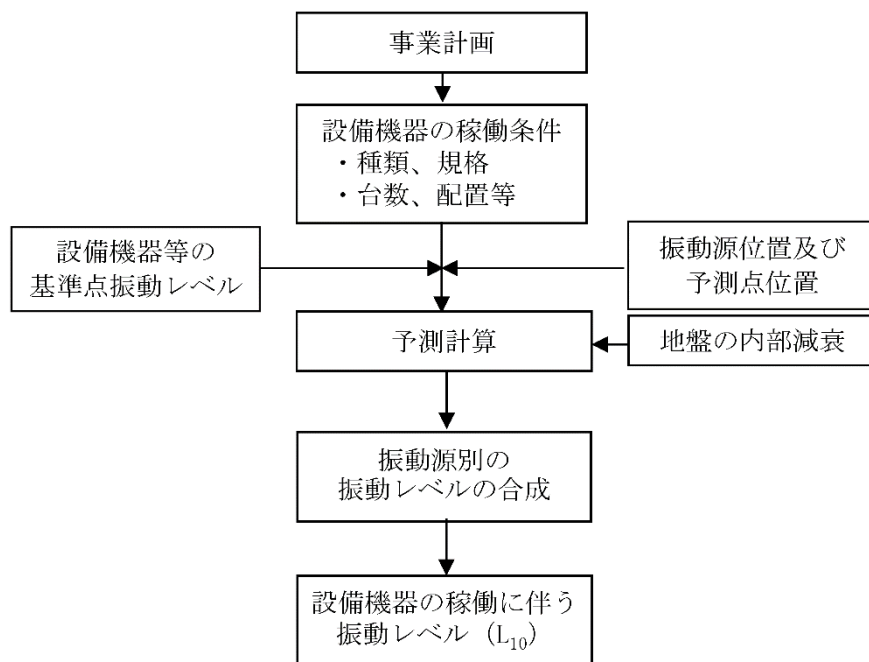
図 5-2-4-5 予測手順（施設の稼働に伴う振動）
