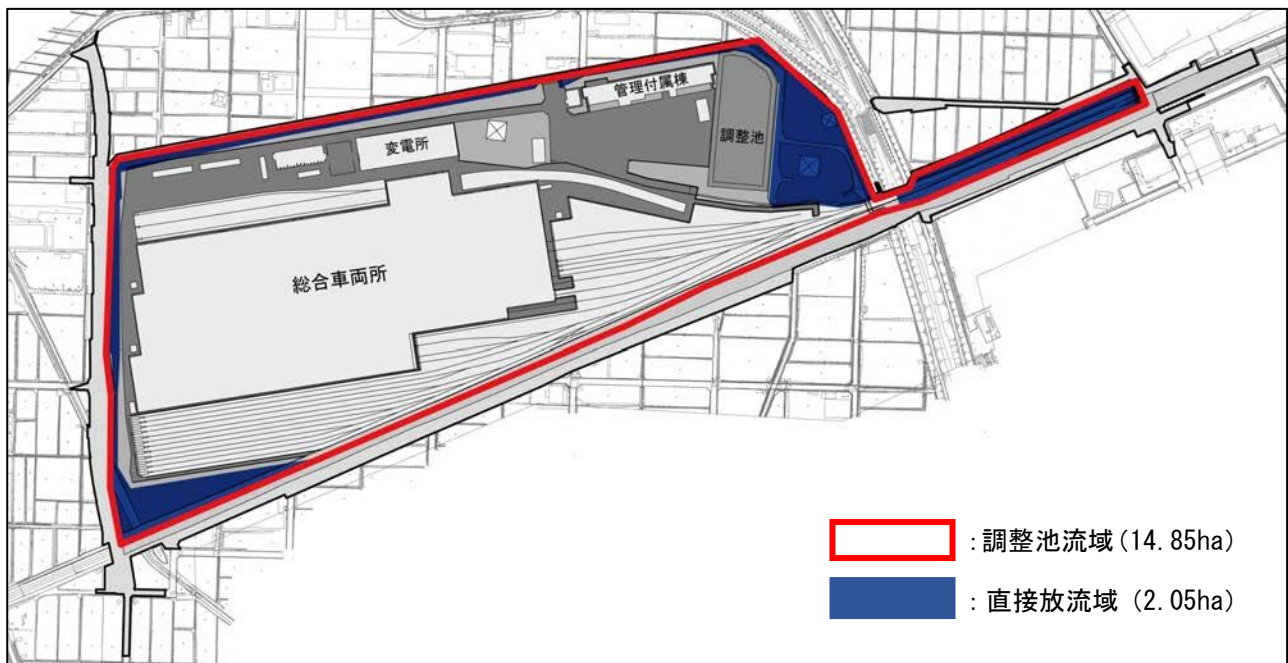
図 5-2-7-1 調整池の流域設定
