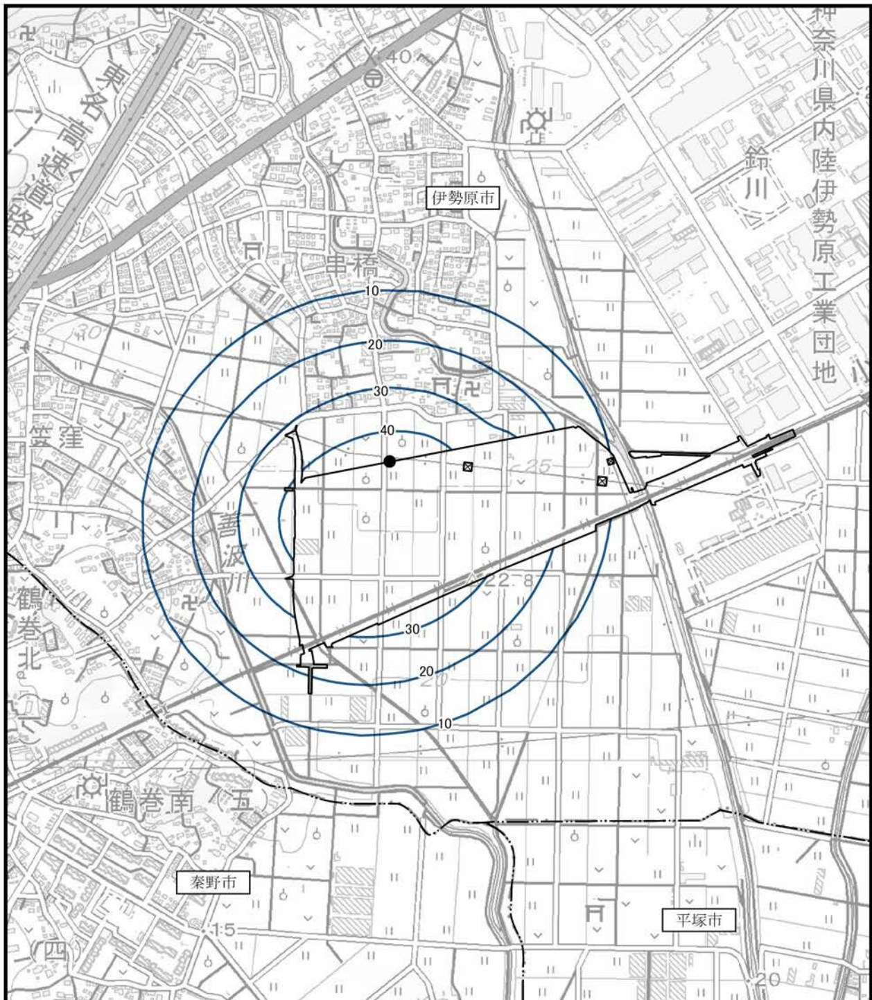
図 5-2-4-7 施設の稼働に伴う振動の予測結果
