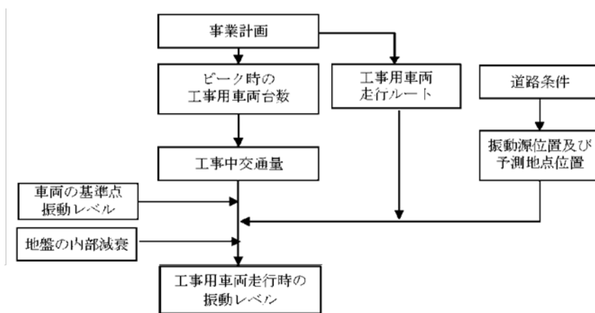
図5-2-4-3(1) 予測手順(工事用車両の走行に伴う振動 (No.1 都市計画道路田中笠窪線))
