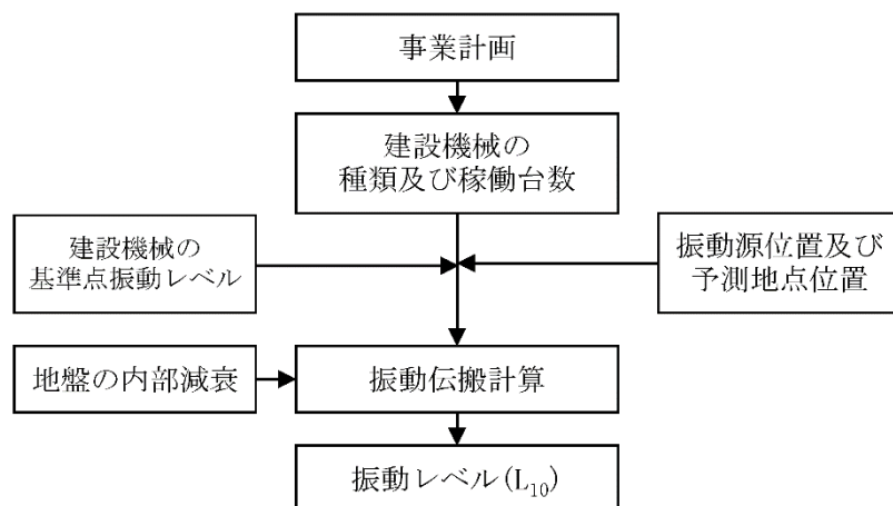
図 5-2-4-1 予測手順（建設機械の稼働に伴う振動）
