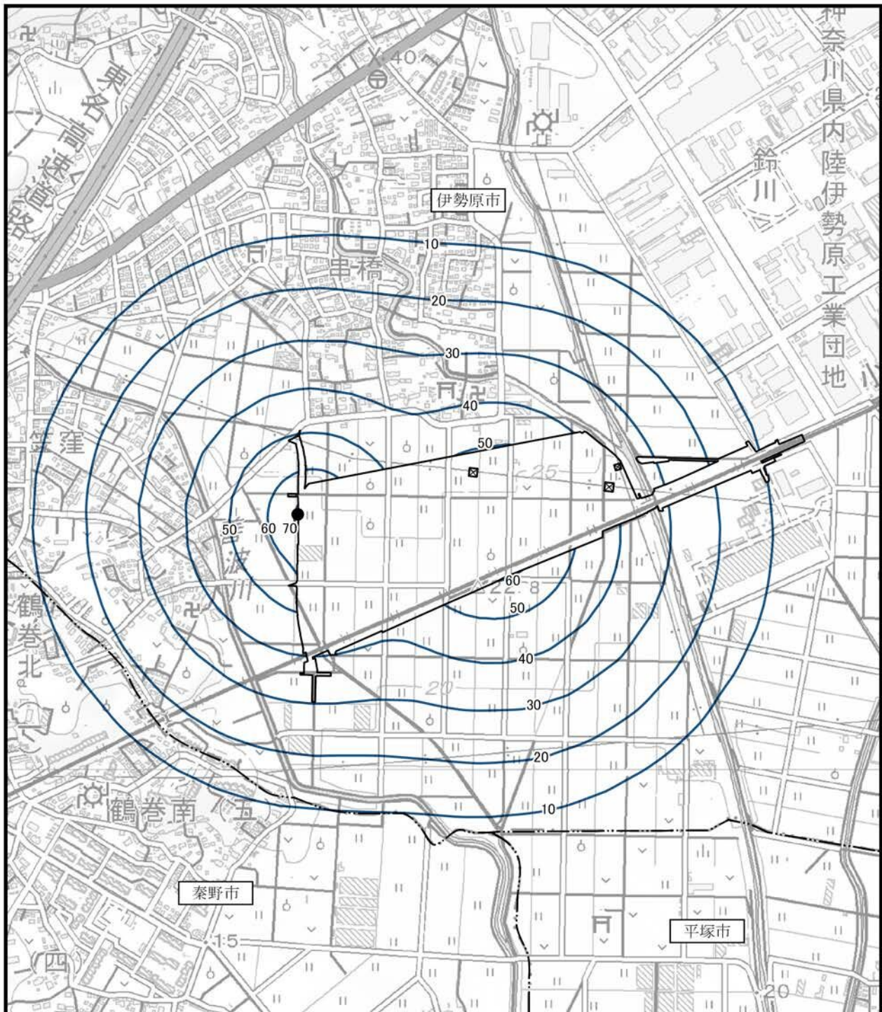
図 5-2-4-2 建設機械の稼働に伴う振動の予測結果
