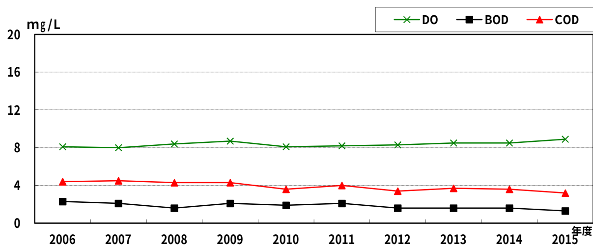
図3-9 金目川 (花水橋)
