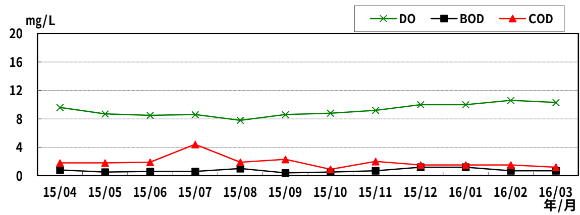
图4-10 酒匂川 (飯泉取水堰 (上))
