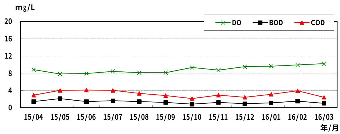
图4-9 金目川 (花水橋)
