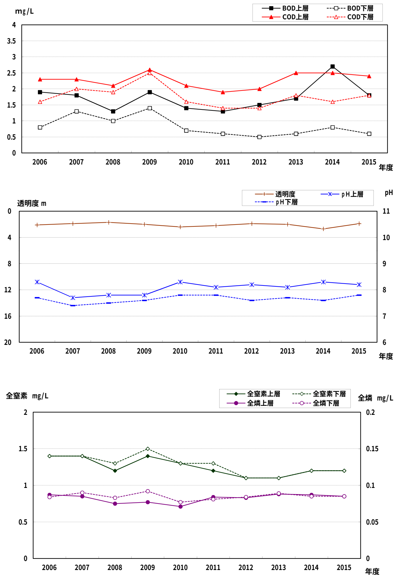
図7－1 相模湖 (湖央東部)
