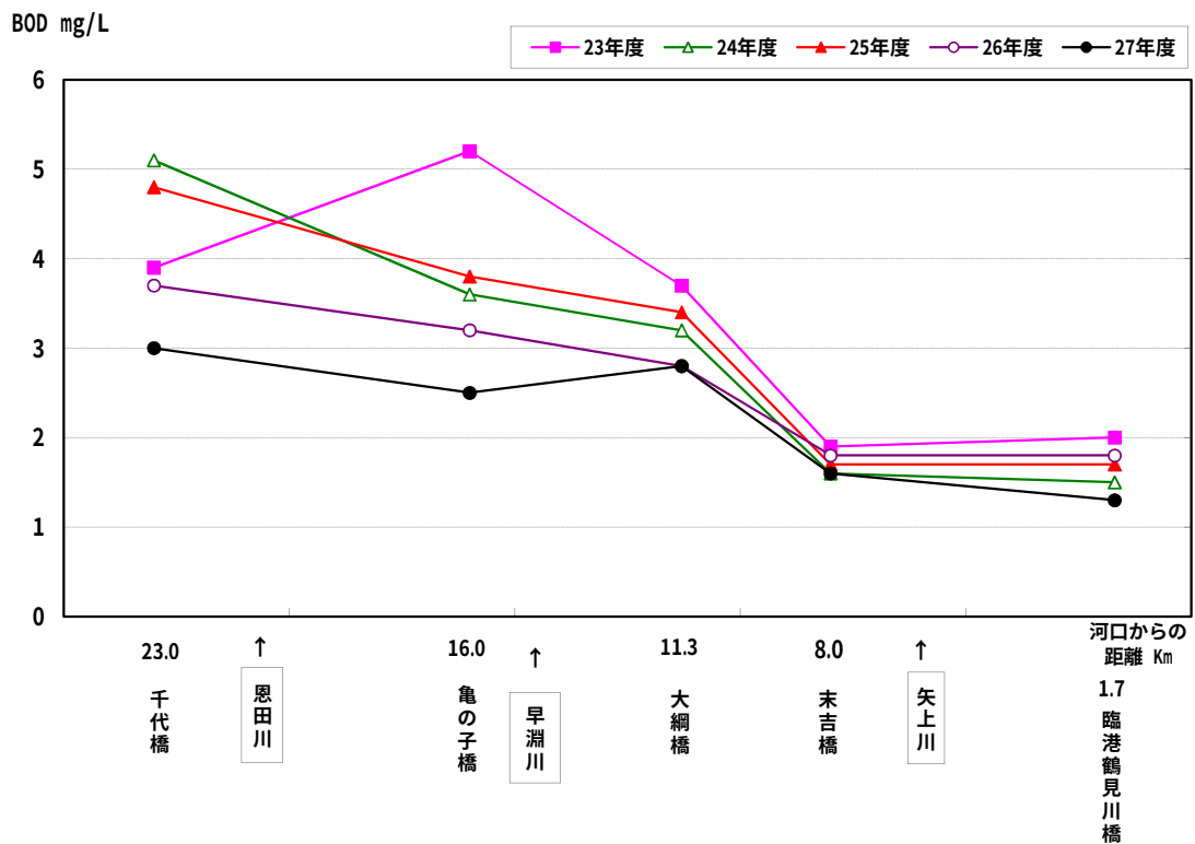
図２－２ 鶴見川におけるBOD縦断変化図
