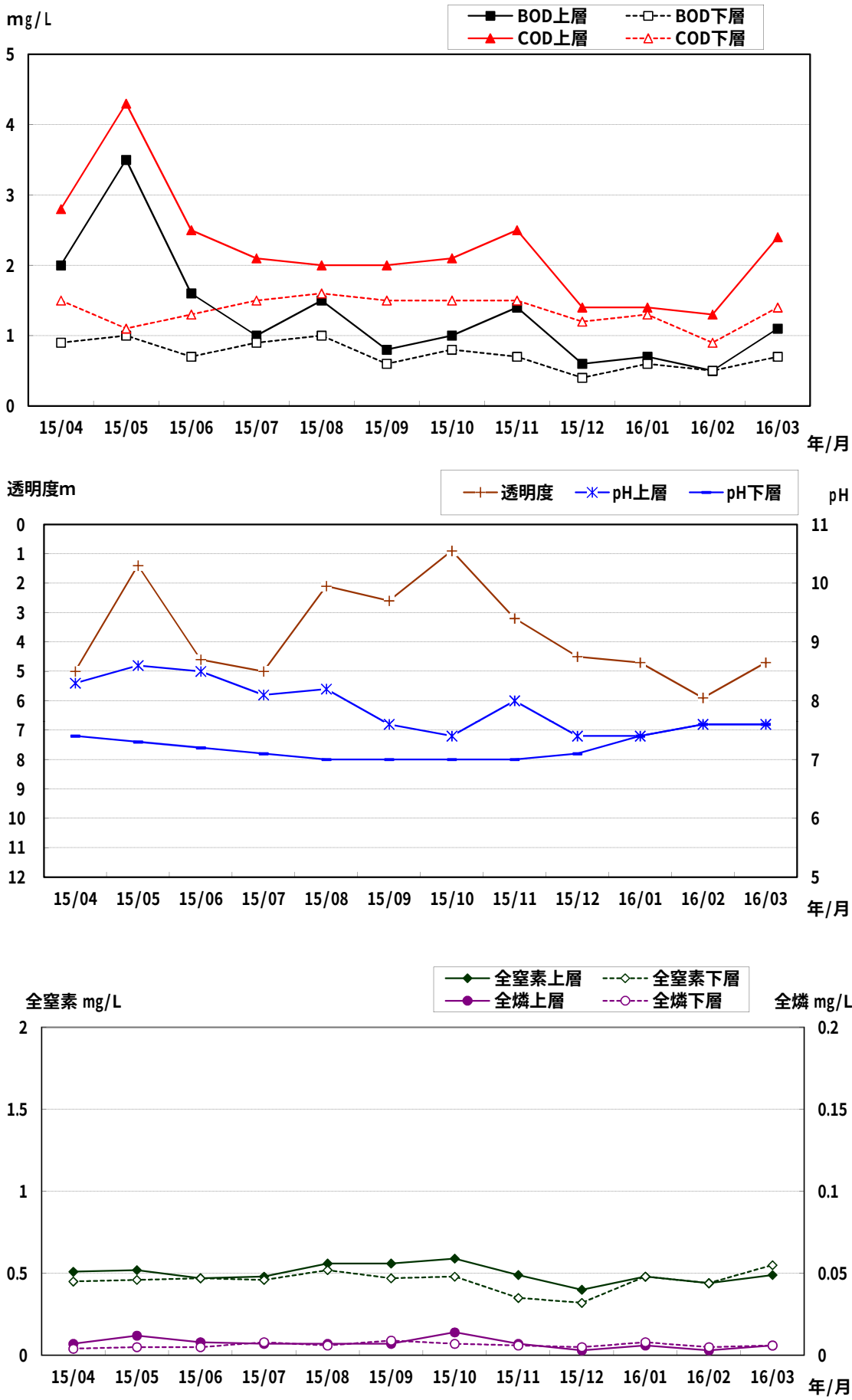
图8-3 丹沢湖(湖央部)
