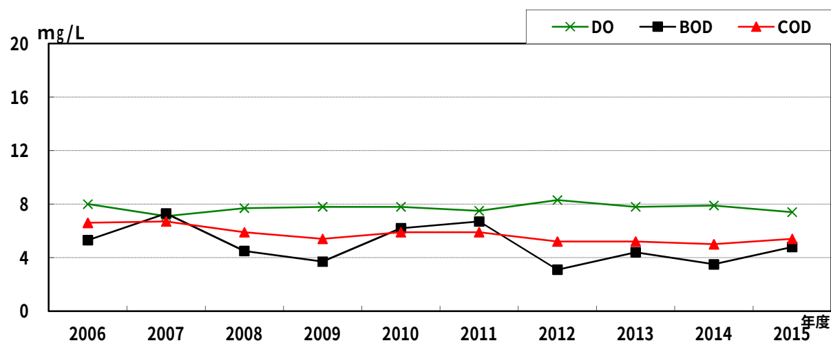
図3-8 相模川 (寒川取水堰 (上))
