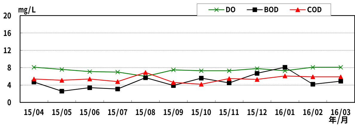
图4-8 相模川 (寒川取水堰 (上))
