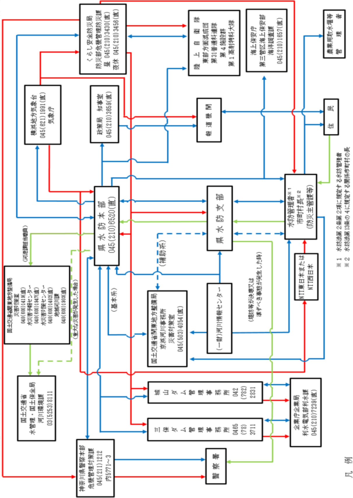
(3)水防時における通信連絡基本系統図 (基本情報連絡関係) [その1]
