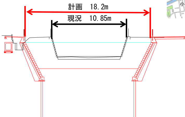
【標準横断図】
