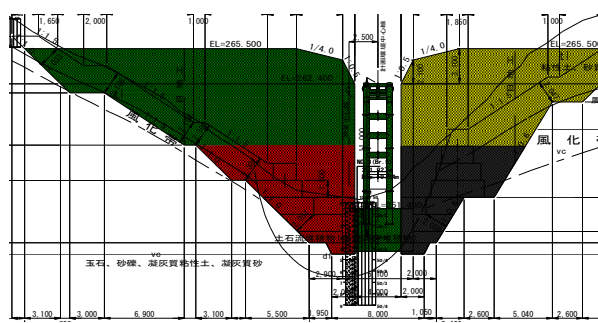
【堰堤工正面図】 （計画-4 堰堤）
