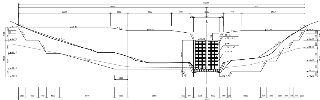
構造図
