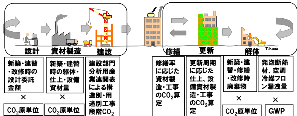
図Ⅲ.2.3 建物のLCA指針におけるCO 2 排出量の積上げ(「建設」「修繕・更新・解体」時)
