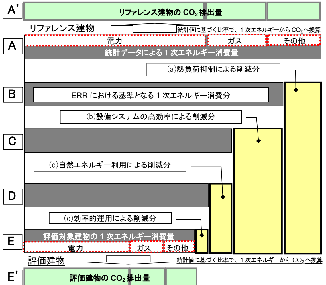
図Ⅲ.2.4 評価対象建物のCO 2 排出量算定の考え方
