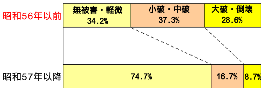
建設時期と地震被害状況 （平成7年阪神・淡路大震災調査委員会中間報告（建設省）より作成）
