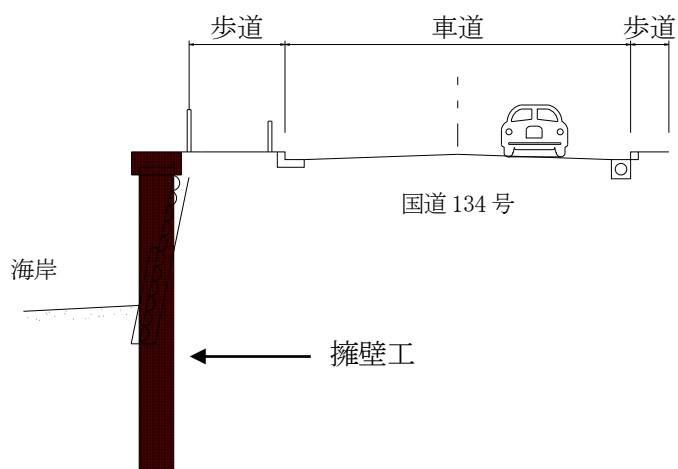
標準横断図
