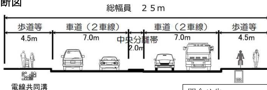
標準横断面図
