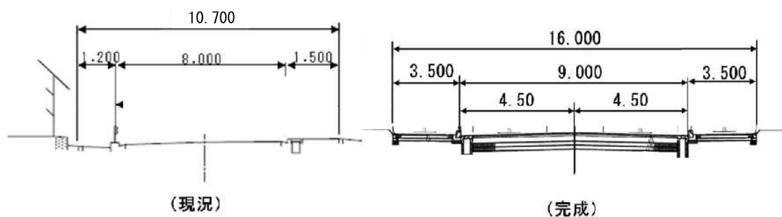
標準断面図
