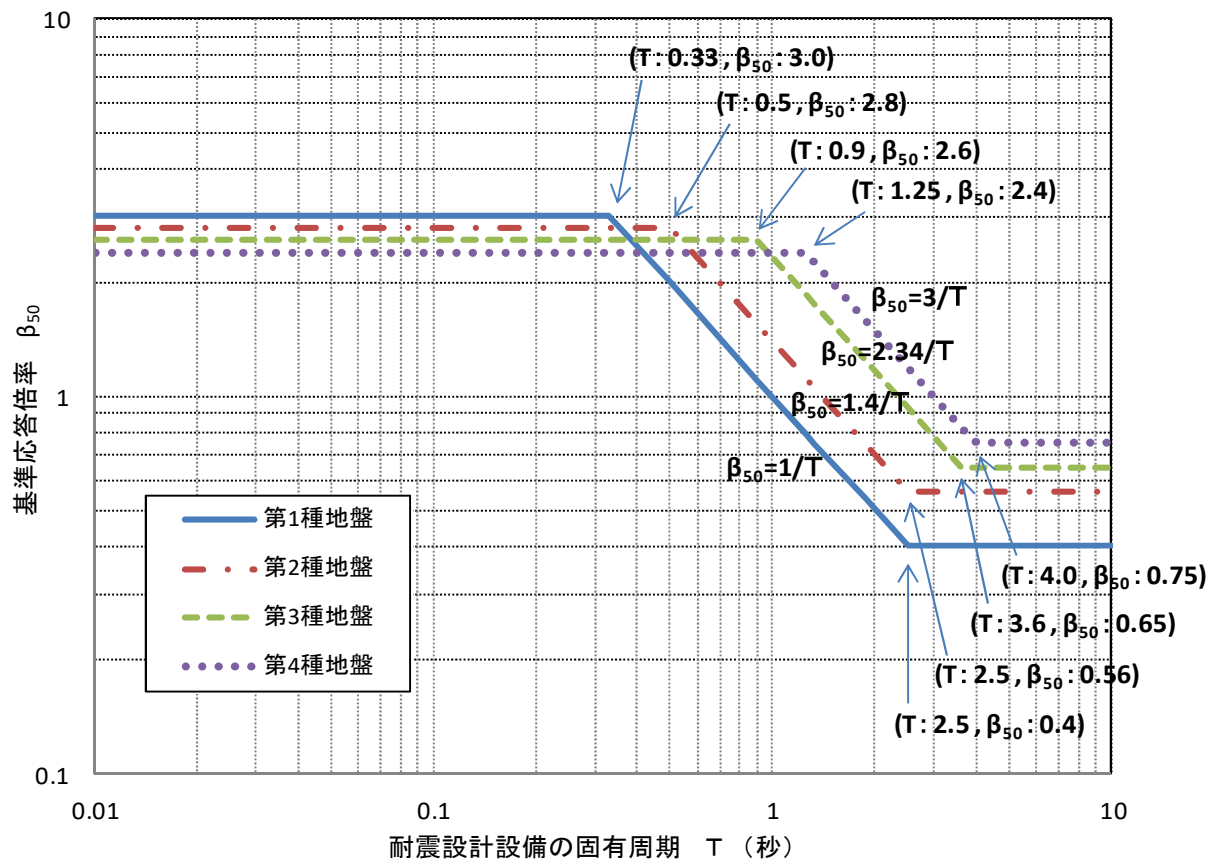
別図 耐震設計設備の標準応答倍率
