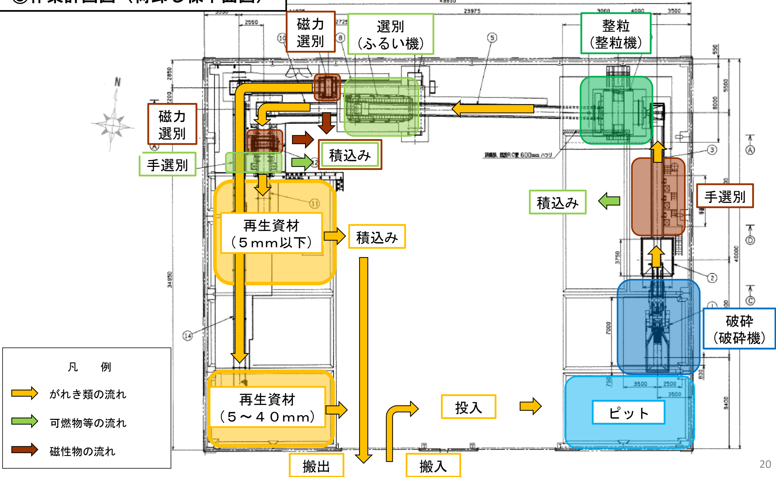
③作業計画図 (荷卸し棟平面図)
