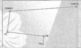
基準点網図 1/2000
