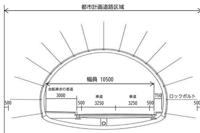
3・6・10号長柄上山口線（幅員10.5m）
