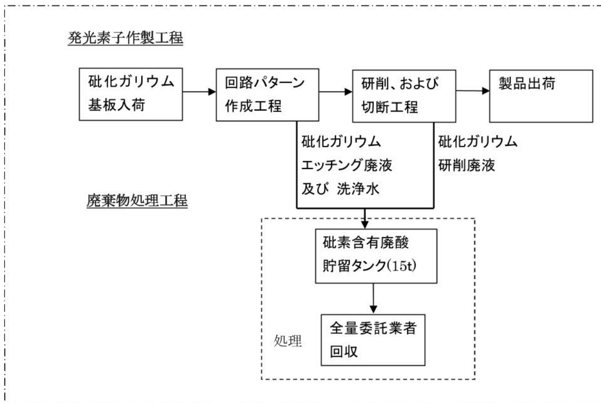
発光素子作製、及び廃棄物発生/処理フロー図
