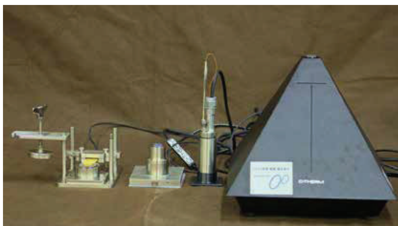
図1：熱伝導率測定装置とセンサー(左から TPSセンサー、mTPSセンサー、液体専用ユニット)
