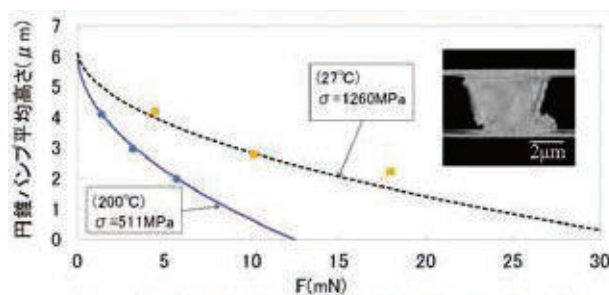
図3：フリップチップ接合試験
