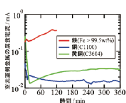
図3：酸素濃淡電池腐食試験中における窒素室側金属の腐食電流の変化
