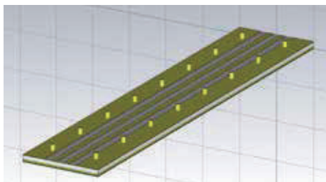
図1：電磁界解析モデル
