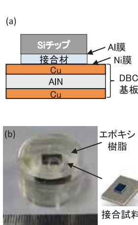
図2：研磨試料 (a) 断面模式図 (b) 試料外観
