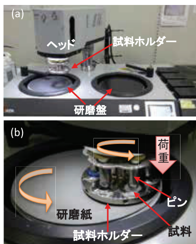
図1：研磨装置外観
