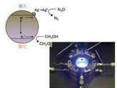
(上)推定反応メカニズムと(下)試験の様子
