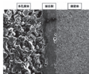
SEM観察による接合界面の状態
