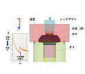
図2 分流鍛造シミュレーション
