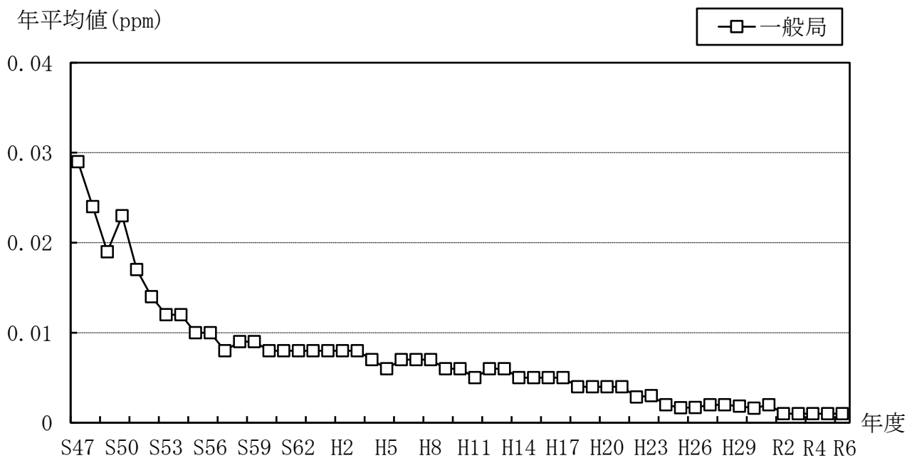
図9 二酸化硫黄(SO 2 )の年平均値の経年推移
