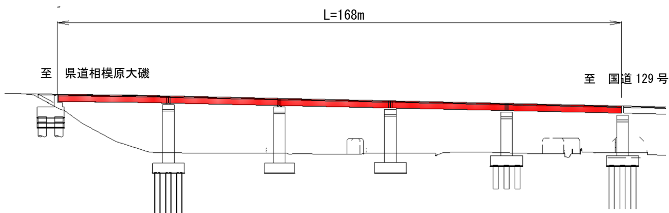
【橋梁側面図】
