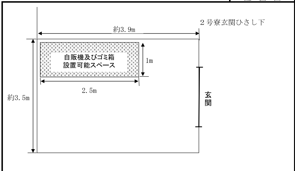
配置図
