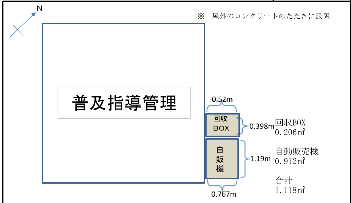
配置図
