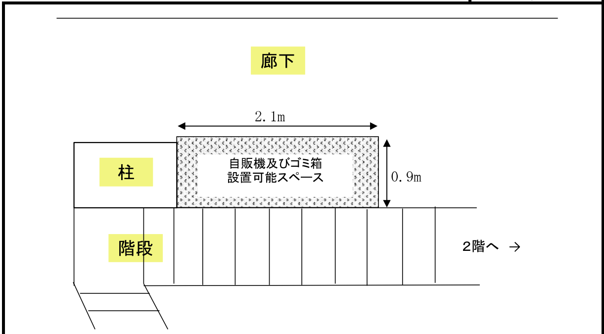
配置図
