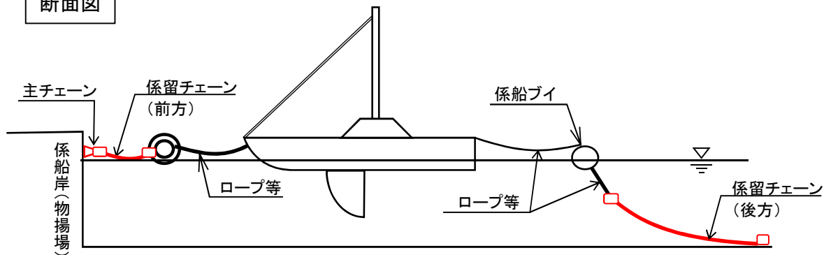
断面図
