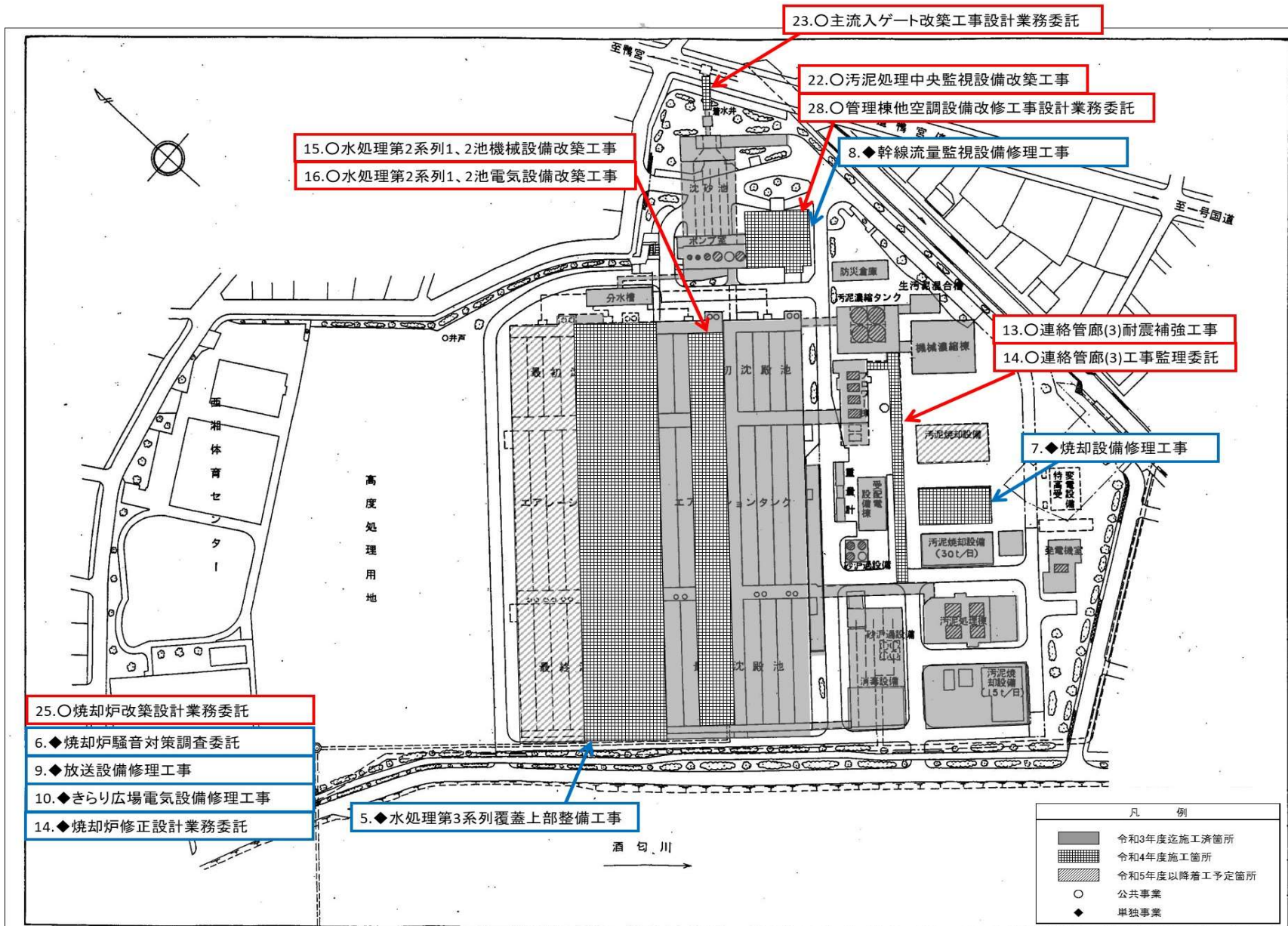
②令和4年度 酒匂川流域下水道 左岸処理場 実施平面図
