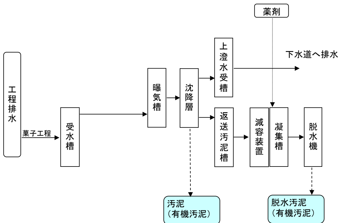
図2 排水処理フローシート〔NO.2〕
